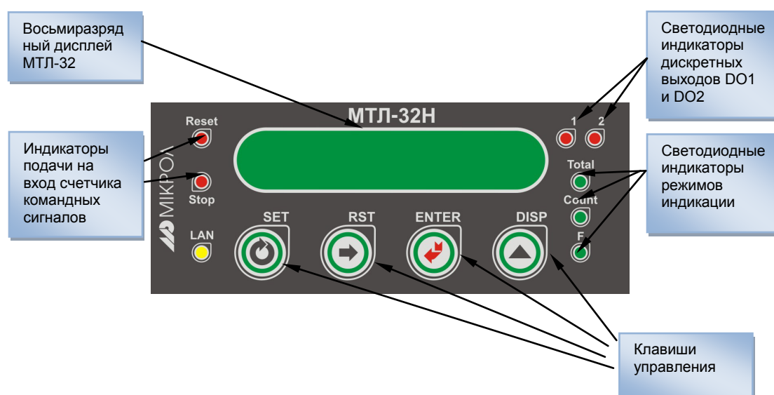
Рисунок 3.1 - Внешний вид передней панели счетчика МТЛ-32Н
