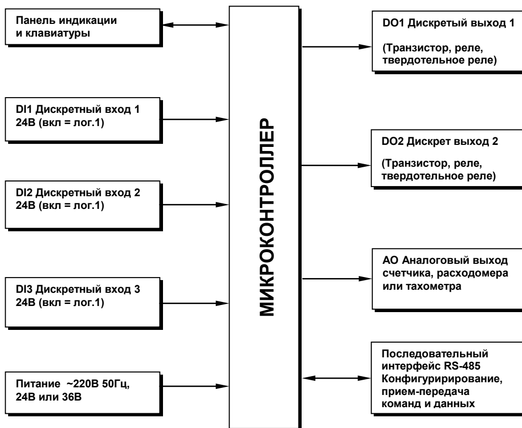
Рисунок 3.2 - Структурная схема счетчика МТЛ-32Н
