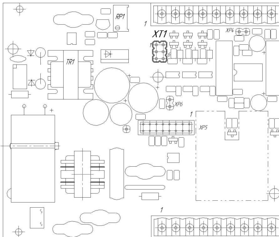
Рисунок Б.1.4 - Расположение перемычек XT1 для настройки дискретных входов
