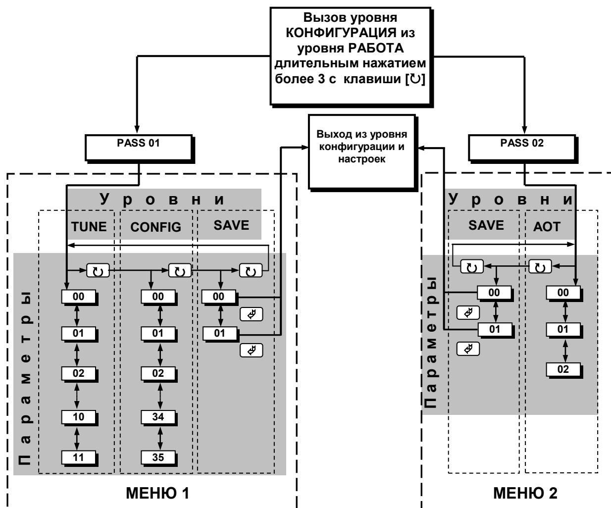
Рисунок 4.2 - Диаграмма уровней конфигурации и настроек.
