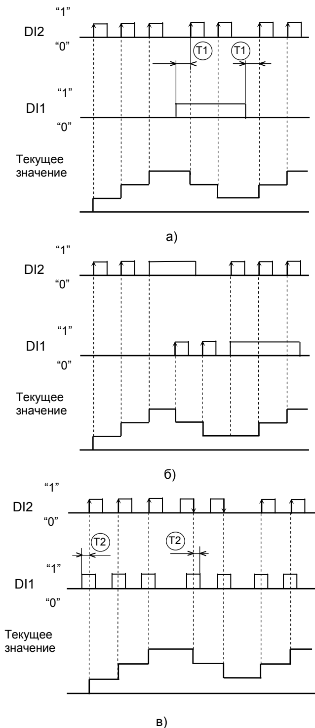
Рисунок 5.2 – Диаграммы работы счетчика МТЛ-32Н в реверсивных режимах счета
