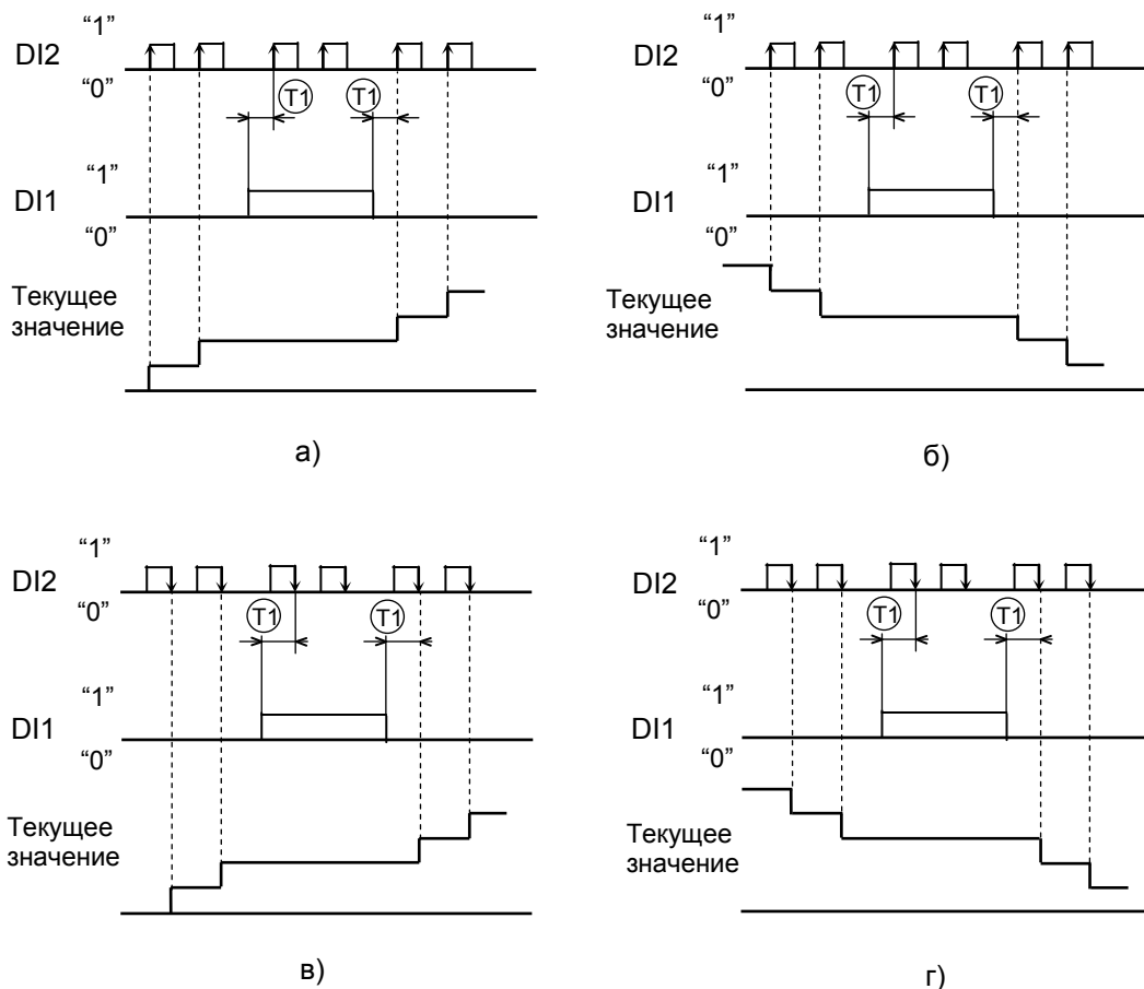
Рисунок 5.1 – Диаграммы работы счетчика МТЛ-32Н в суммирующем и вычитающем режимах счета
