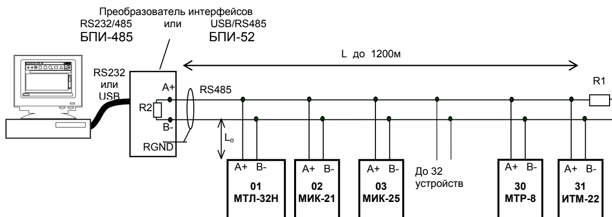
Рисунок Б.2 - Организация интерфейсной связи между компьютером и контроллерами
