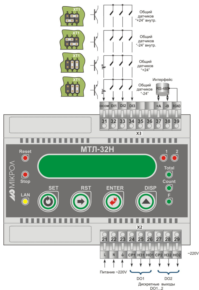
Рисунок Б.1.1 - Подключение внешних цепей счетчика МТЛ-32Н. Исполнение на напряжение 220 В переменного тока
