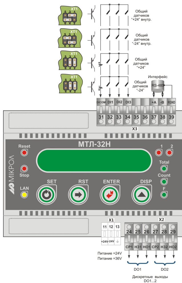
Рисунок Б.1.3 - Подключение внешних цепей счетчика МТЛ-32Н. Исполнение на напряжение 24 В постоянного тока
