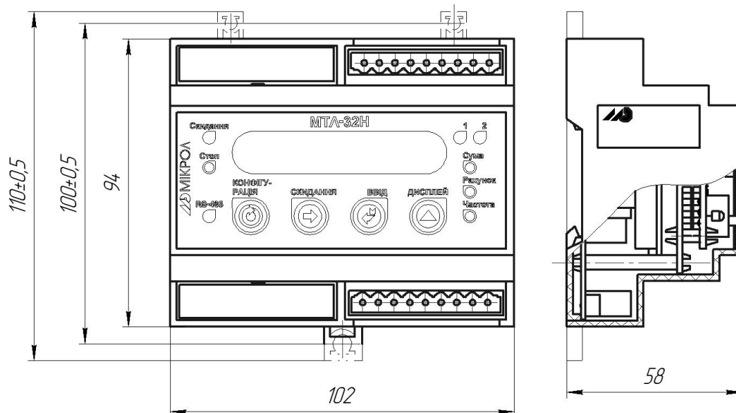
Рисунок А.2 - Габаритные размеры
