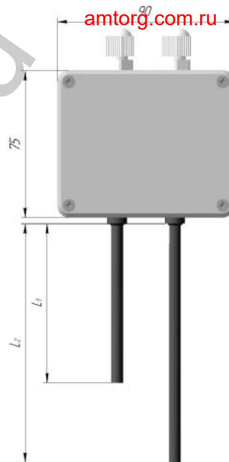
Рисунок 2 – Габаритно-установочные размеры
