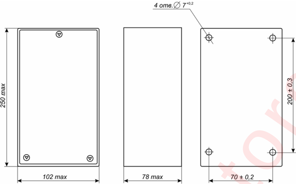
Рисунок 1 – Габаритные и присоединительные размеры паркового переговорного устройства ППУ.М2
