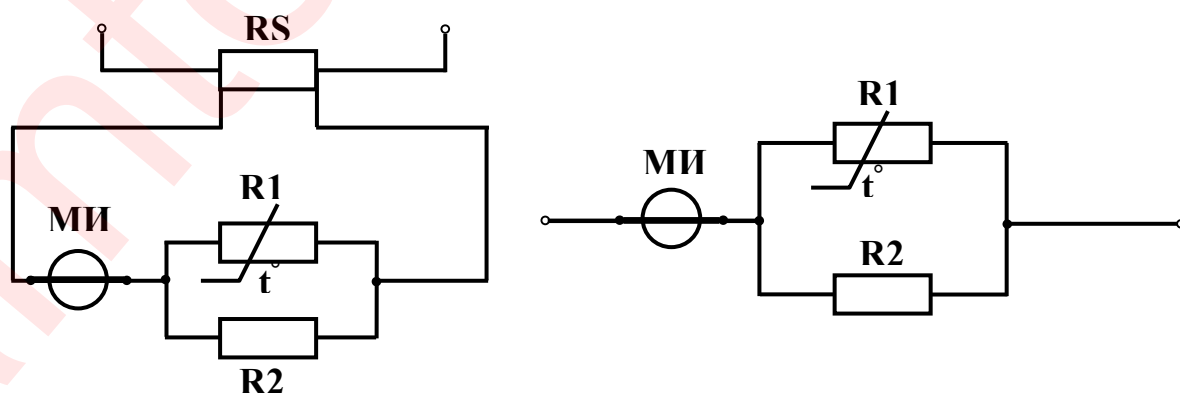
Рис.1 Схемы электрические принципиальные амперметров М1420 и М1420.1
