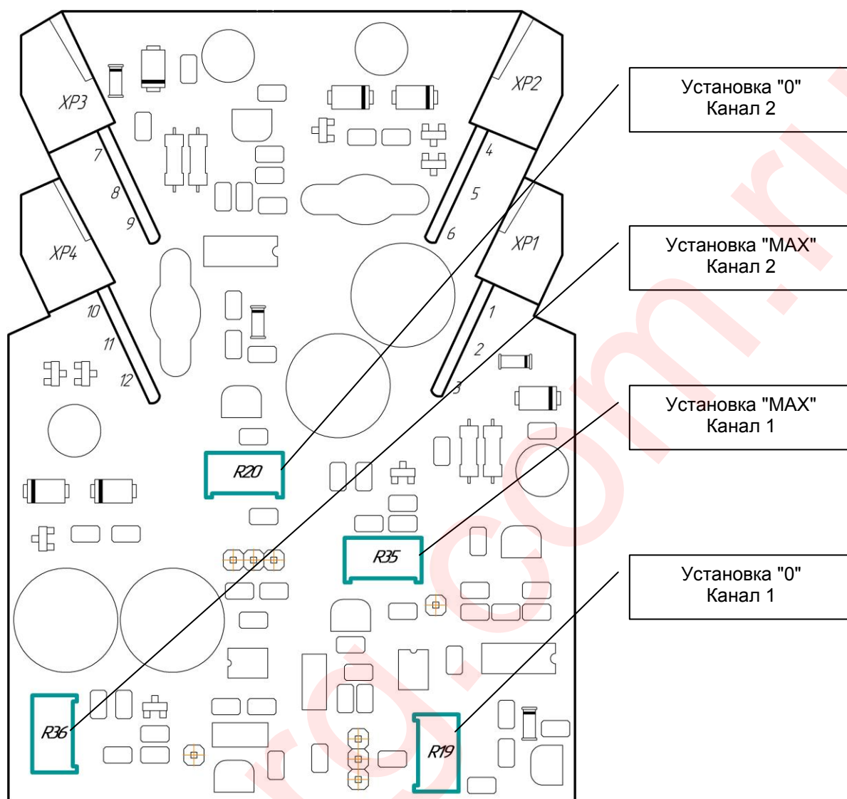
Рисунок 4.1 – Схема расположения элементов настройки БРГ-412
