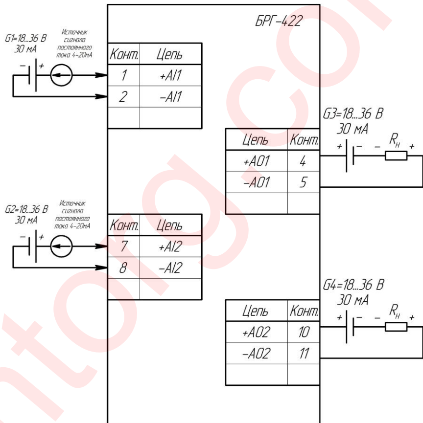
Рисунок 3.2 – Схема электрических подключений
