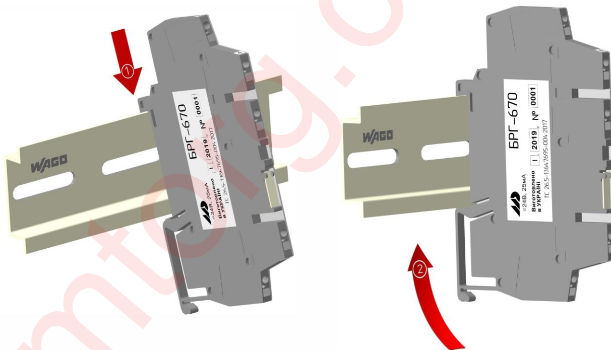
Рисунок 3.2 – Схема крепления блока BRG-670 на DIN-рейку
