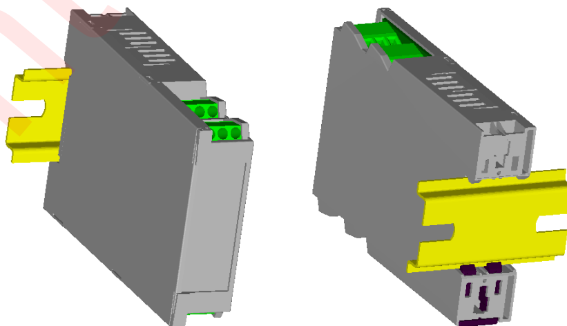
Рисунок 3.2 – Схема крепления блока БПО-430/БПО-432 на DIN-рейку
