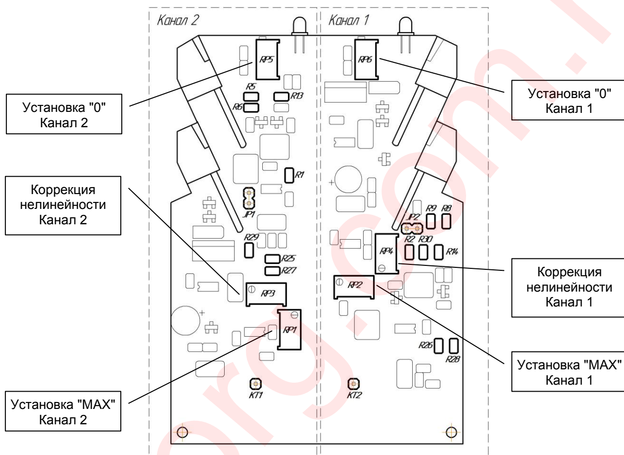
Рисунок 3.1 – Схема расположения органов регулирования и элементов настройки блоков БПО-430/БПО-432
