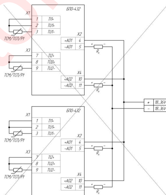
Рисунок 3.5 – Запрещенная схема электрических подключений блока БПО-430/БПО-432
