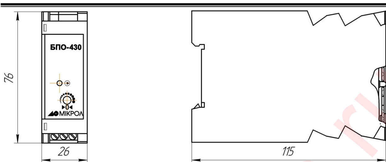
Рисунок 1.1 – Внешний вид и габаритные размеры БПО-430
