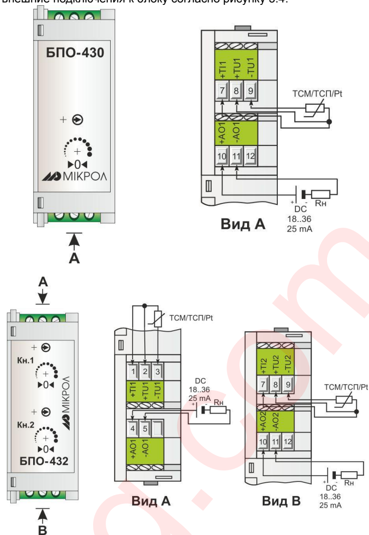
Рисунок 3.4 – Схема электрических подключений блока БПО-430/БПО-432
