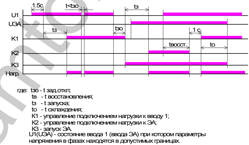
Рис.6 Временные диаграммы включения и отключения ЭА при пропадании и появлении напряжения на вводе 1
