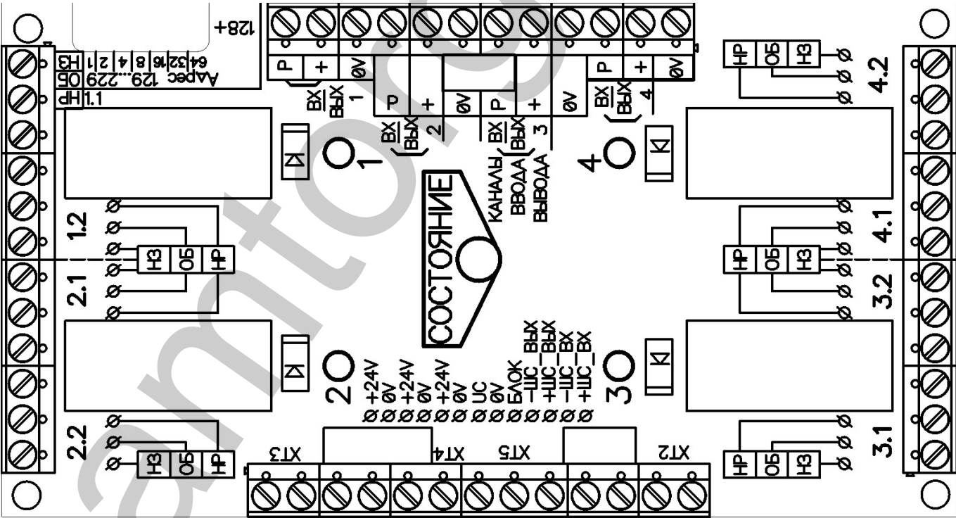
Внешний вид и расположение клемм БВВ-А-01
