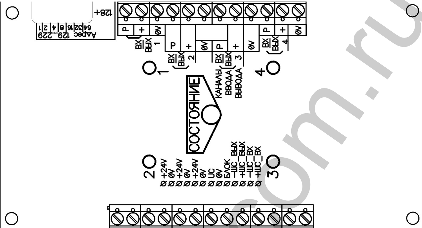
Внешний вид и расположение клемм БВВ-А, БВВ-А-02
