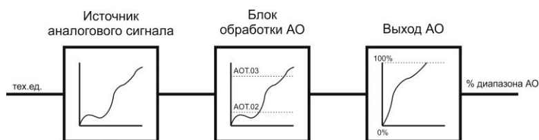
Рисунок 3.6 – Работа блока аналогового выхода в режиме ретрансмиссии
