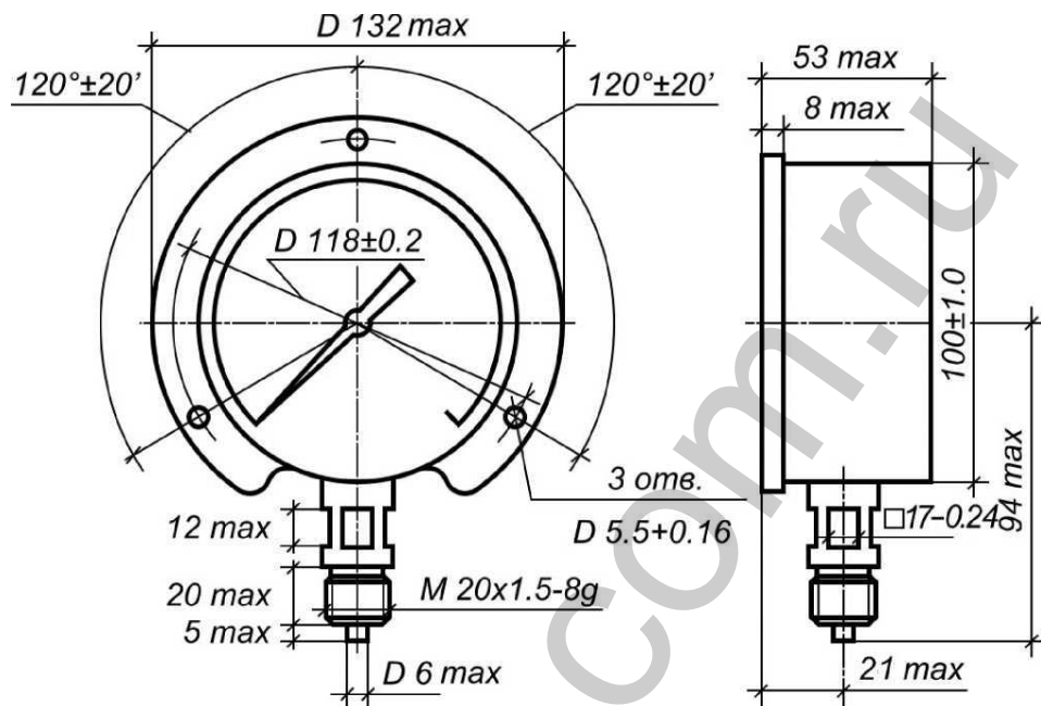
Габаритные и присоединительные размеры МП-У2
