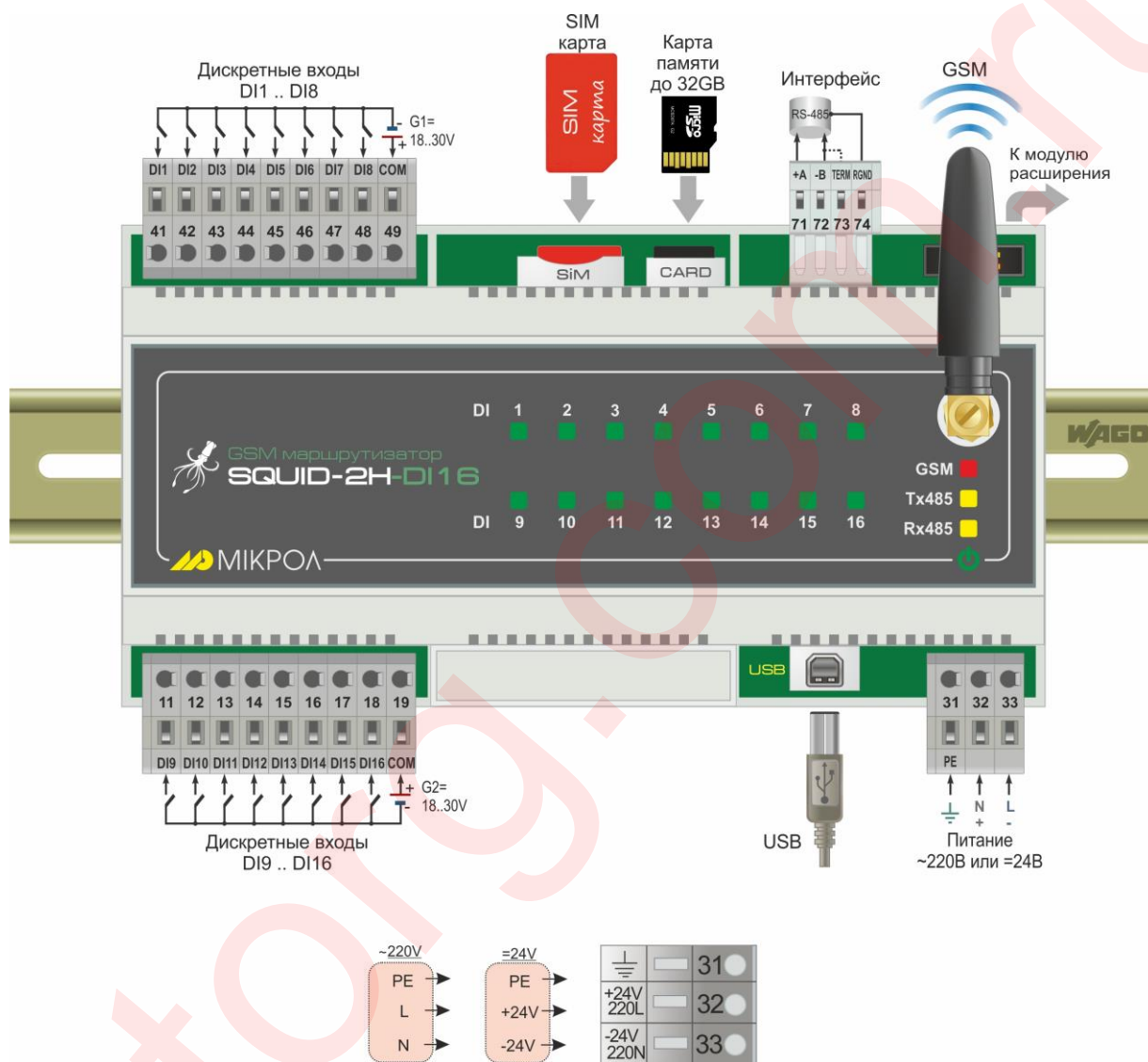
Рисунок А.2 – Расположение внешних соединительных устройства SQUID-2H-DI16
