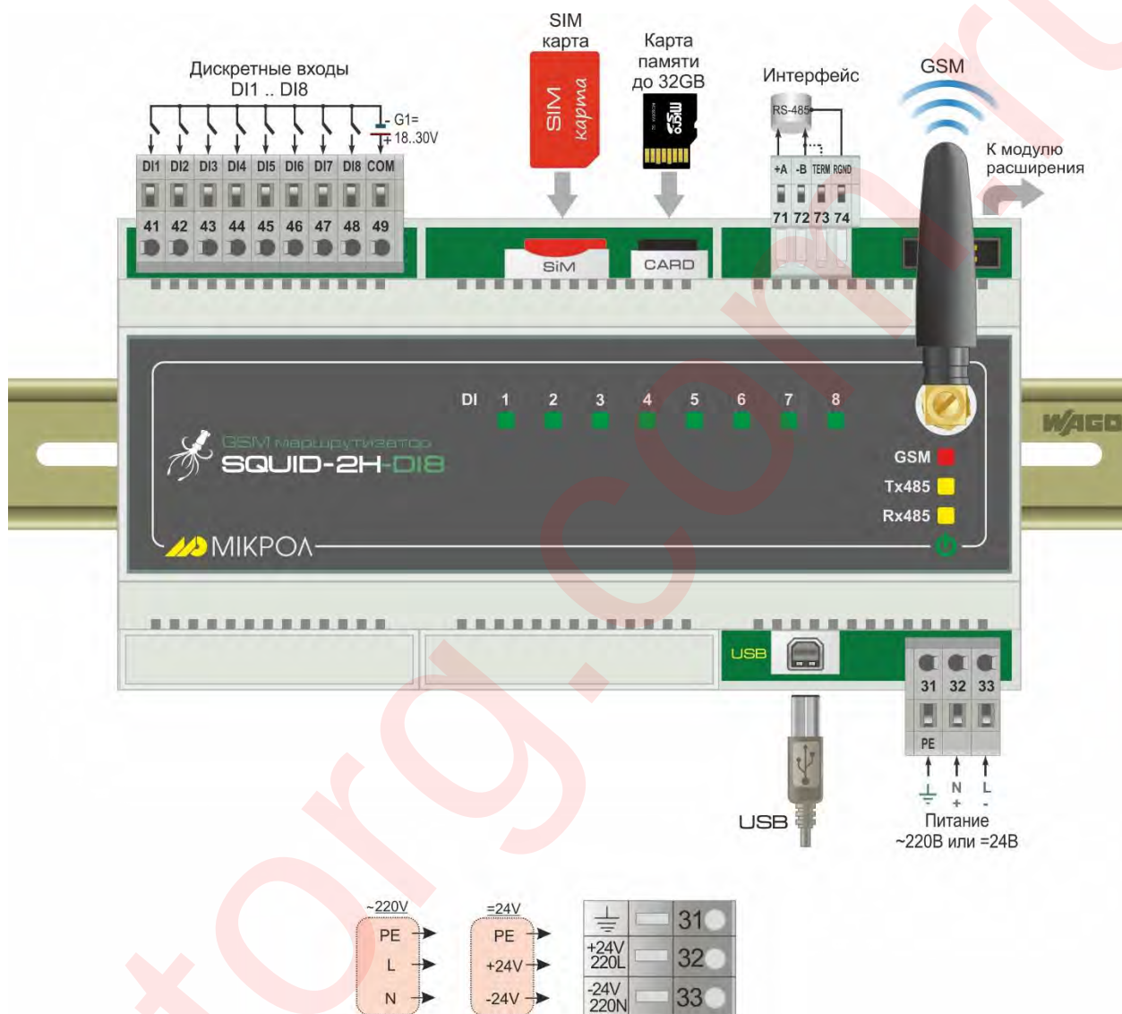
Рисунок А.2 – Расположение внешних соединительных устройств SQUID-2H-DI8
