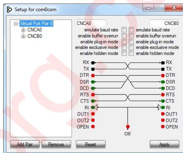
Рисунок 8.1 - Окно настроек программы «com0com»
