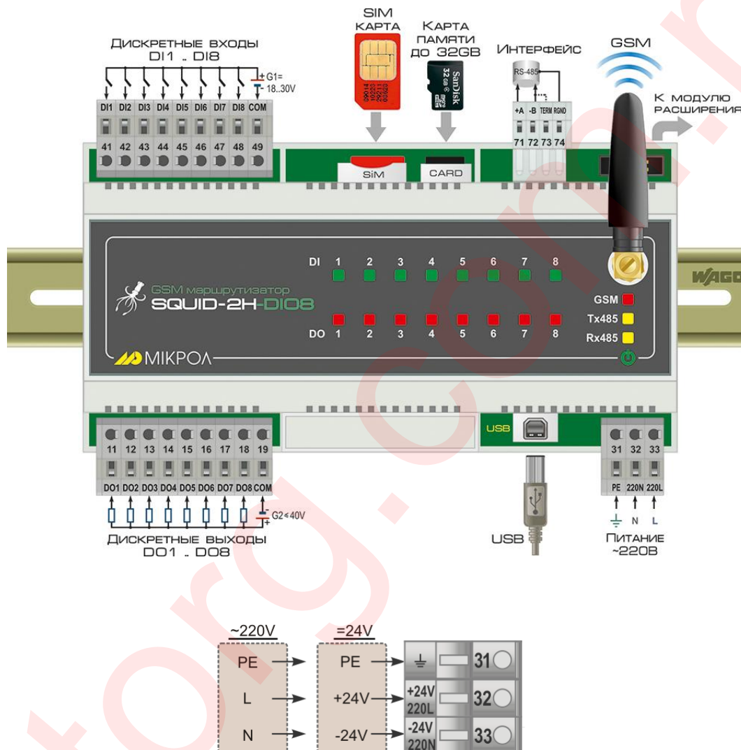
Рисунок А.2 – Расположение внешних соединительных устройства SQUID-2H-DIO8
