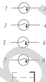
Схема электрическая
