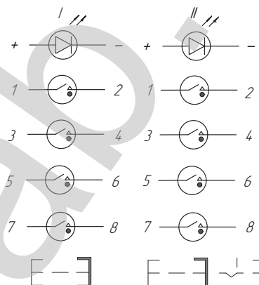
Схема электрическая
