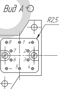
Разметка для крепления
