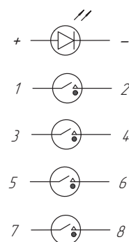
Схема электрическая
