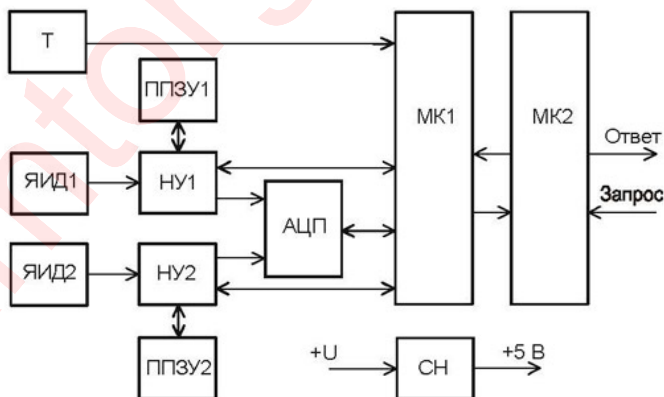
Рисунок 2 – Структурная схема плотномера
