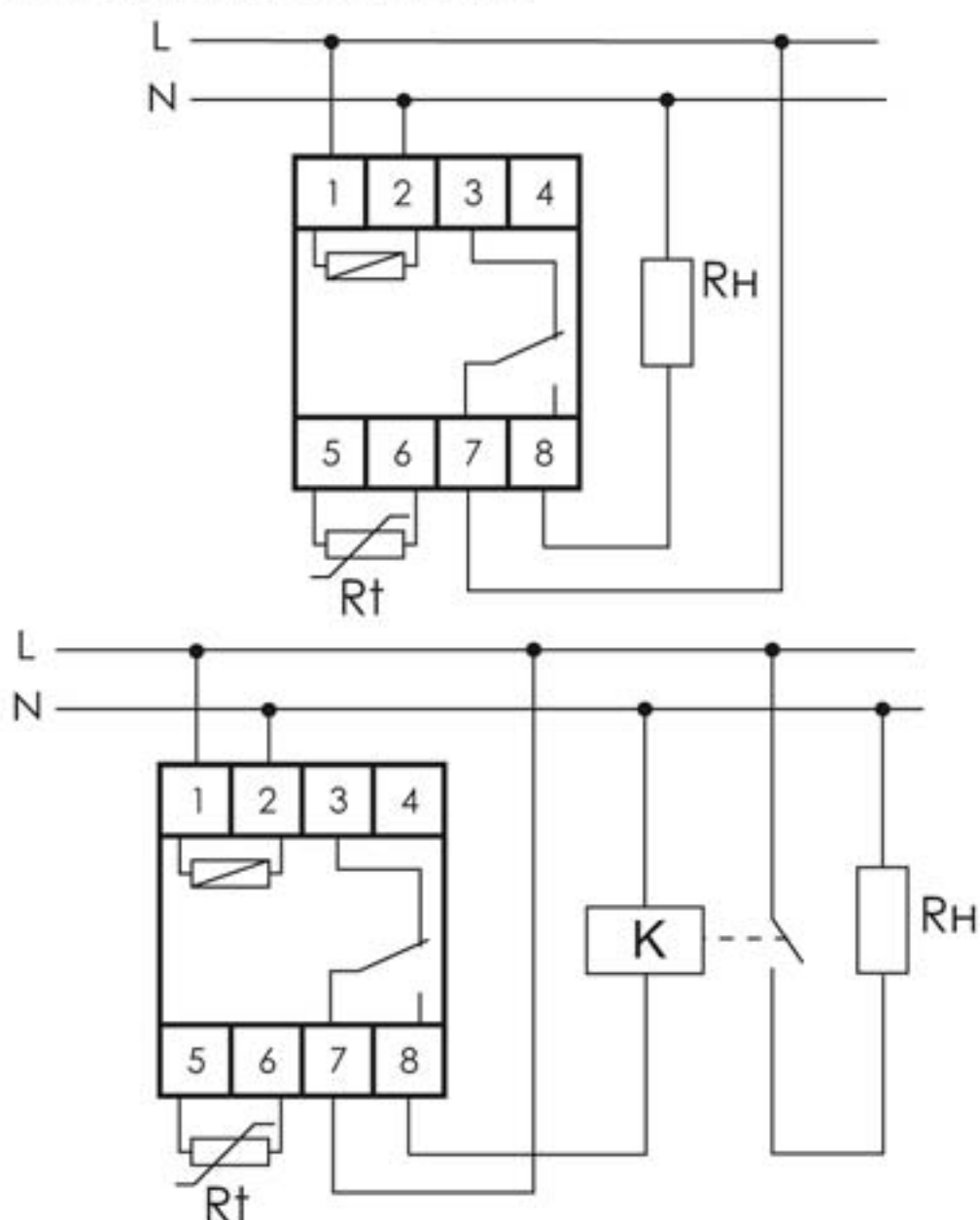
Схема подключения с применением контактора
