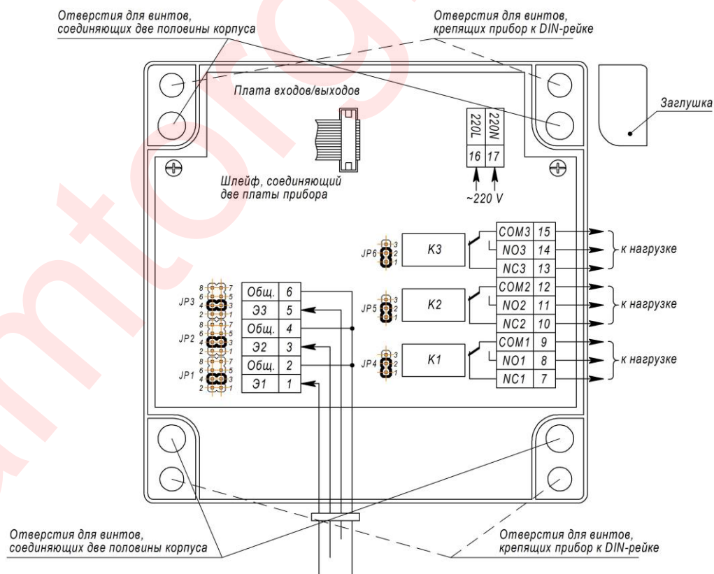
Рисунок 4.2 – Схема подключения внешних сигналов к плате входов/выходов PCY-31
