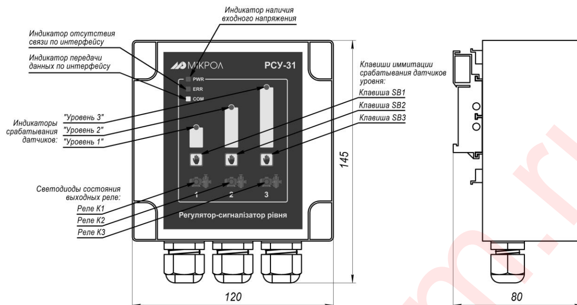
Рисунок 1.4 – Внешний вид и габаритные размеры PCY-31
