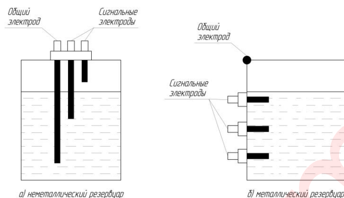
Рисунок 2.1 – Схема размещения электродов в резервуаре
