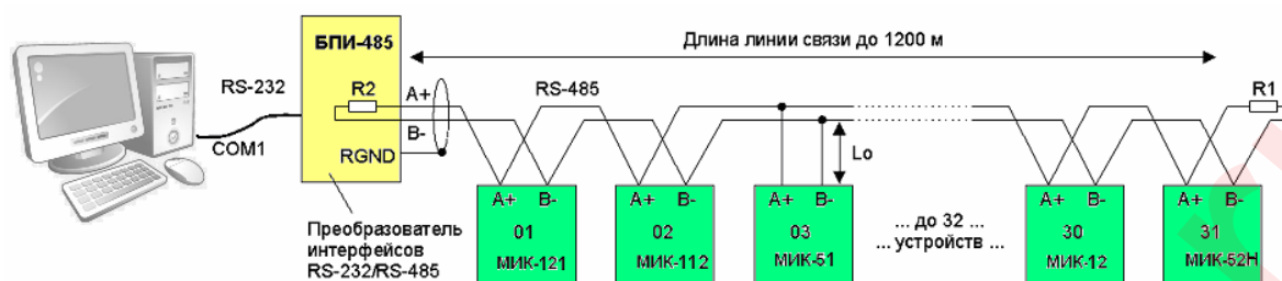
Рисунок Б - Организация интерфейсной связи между компьютером и регуляторами
