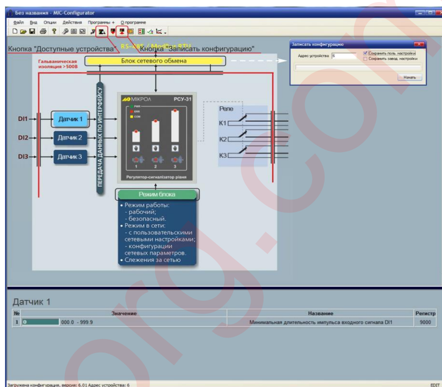
Рисунок 4.5 – Редактирование конфигурации
