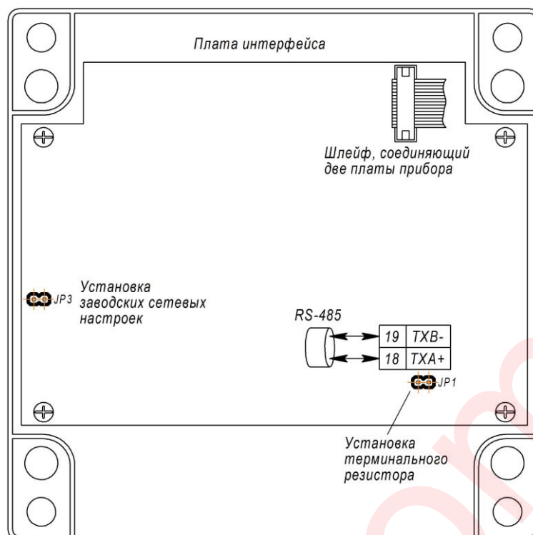
Рисунок 4.3 – Схема подключения внешних сигналов к плате интерфейса РСУ-31
