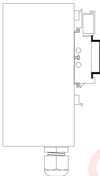
Рисунок 4.1 – Схема установки и снятия блока PCY-31
