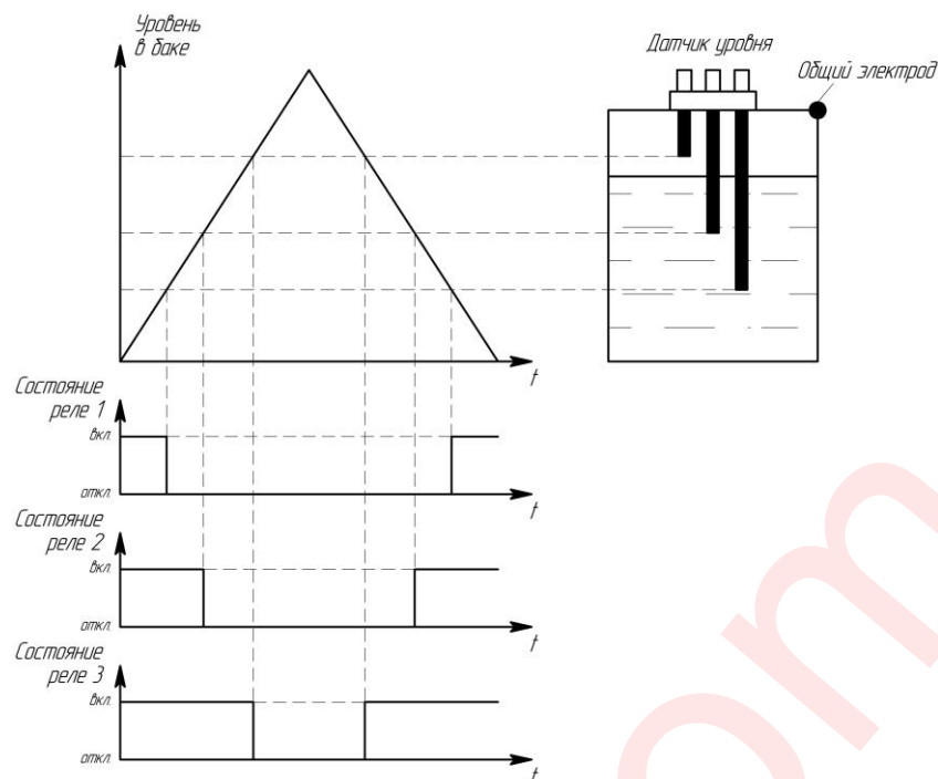
Рисунок 2.3 – Диаграмма работы блока PCY-31
