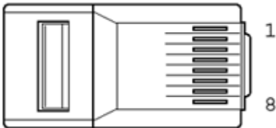
Рисунок А4 – Схема расположения выводов разъема RJ-45 (вид со стороны контактов)
