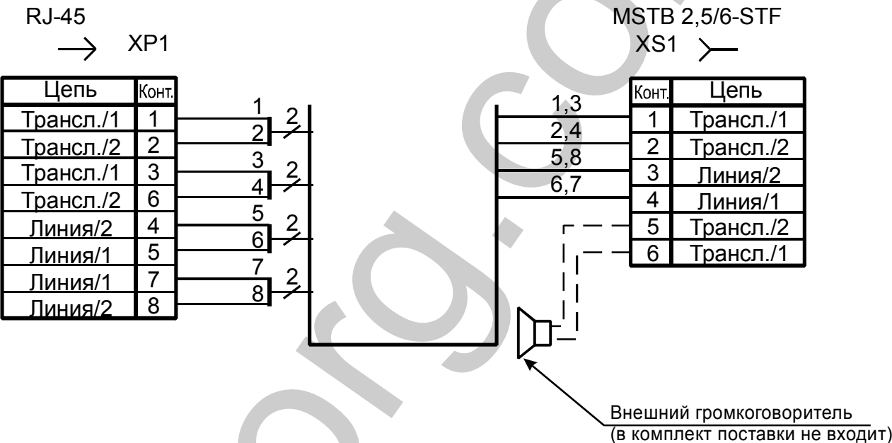
Рисунок А3 – Схема монтажа линий абонента (установка разъемов RJ-45 и MSTB 2,5/6-STF)
