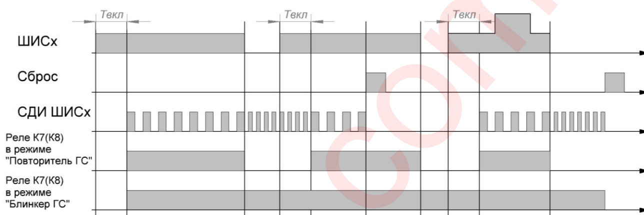
Рисунок 5 – Диаграмма работы датчиков групповой аварийной сигнализации
