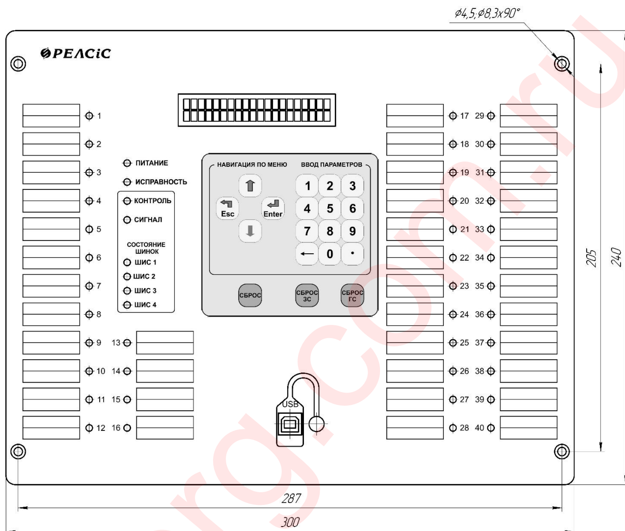
Рисунок А.1 - Габаритные размеры и установочные размеры и внешний вид передней панели устройства РЗЛ-05.Ш1 ЦС
