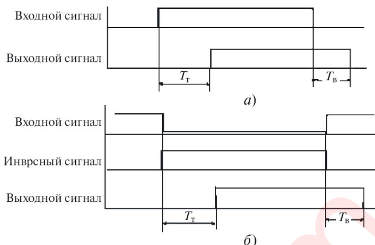
Рисунок 1 – Диаграмма работы дискретного входа 3К (а) и 1К (б)
