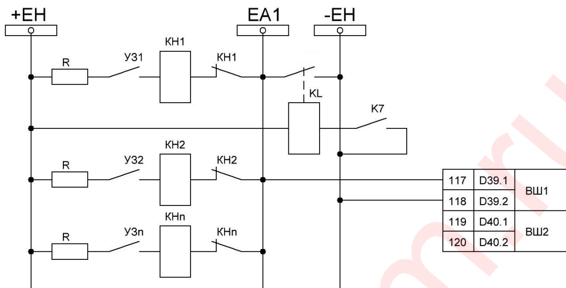
Рисунок 6а – Схема подключения датчиков к вспомогательным шинкам ВШ1, ВШ2
