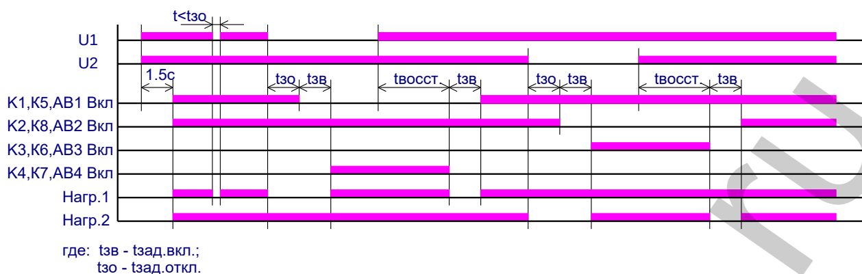
Рис.6 Схема и временные диаграммы работы АВР на автоматических выключателях с двумя равнозначными вводами, двумя группами равнозначных нагрузок, с двумя секционными автоматическими выключателями, с электрической блокировкой секционных автоматических выключателей, с блокировкой при перегрузке по току и управлением от БУАВР.2С.220.220.Т.
