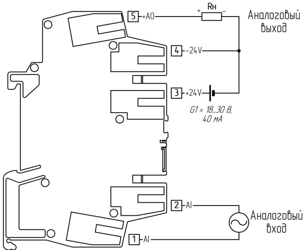
Рисунок 3.4 - Схема внешних соединений преобразователя ПНС-653
