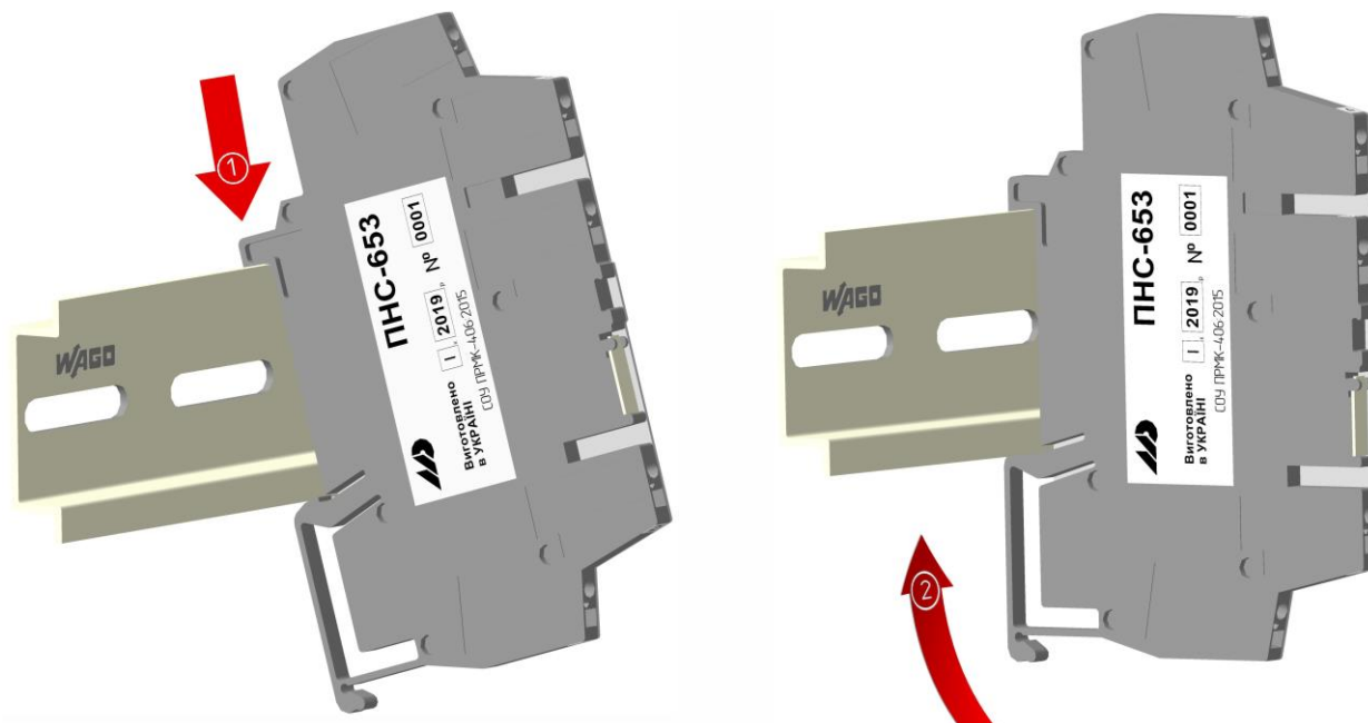
Рисунок 3.2 – Схема крепления преобразователя ПНС-653 на DIN-рейку
