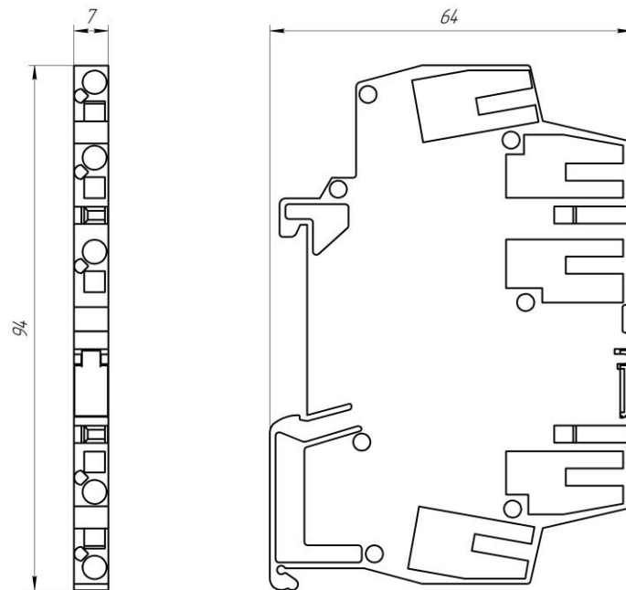
Рисунок 1.1 – Внешний вид и габаритные размеры преобразователя ПНС-653
