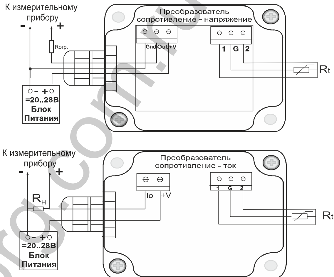
Рисунок 5.2 – Схема внутренних соединений ПТУ-ТСМ(Π)У-012
