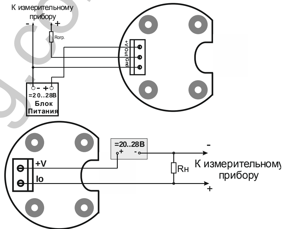
Рисунок 1.2 – Схема внутренних соединений ПТУ-ТСМ(П)У-0016
