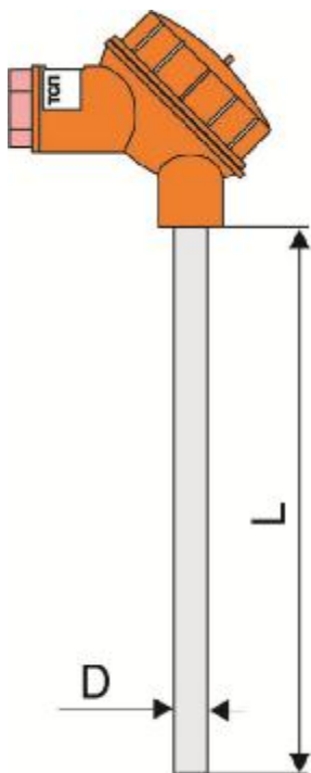
Рисунок 1.1 – Габаритно-установочные размеры ПТУ-ТСМ(П)У-0016
