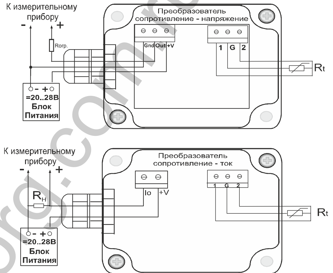
Рисунок 6.2 – Схема внутренних соединений ПТУ-ТСМ(Π)У-303
