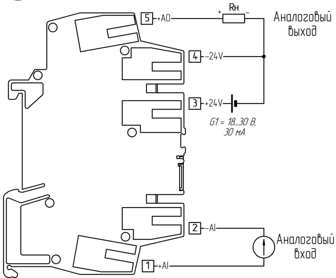
Рисунок 3.4 - Схема внешних соединений преобразователя ПНС-650
