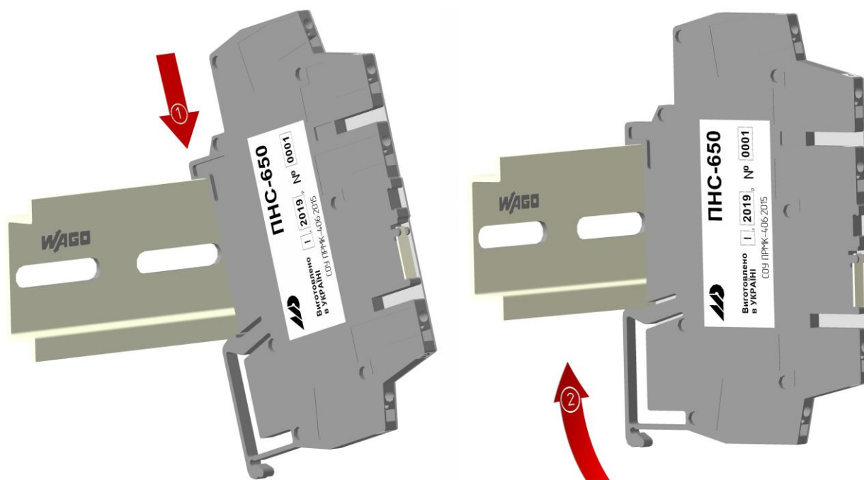
Рисунок 3.2 – Схема крепления преобразователя ПНС-650 на DIN-рейку
