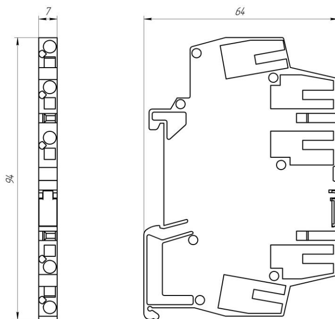
Рисунок 1.1 – Внешний вид и габаритные размеры преобразователя ПНС-651
