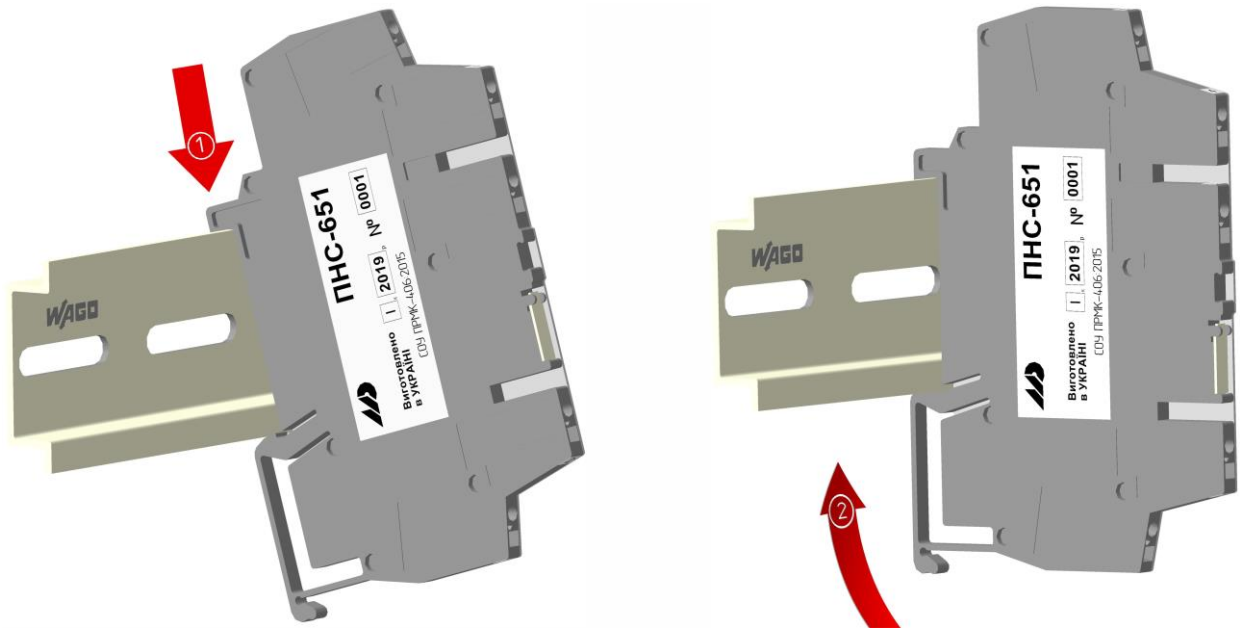
Рисунок 3.2 – Схема крепления преобразователя ПНС-651 на DIN-рейку
