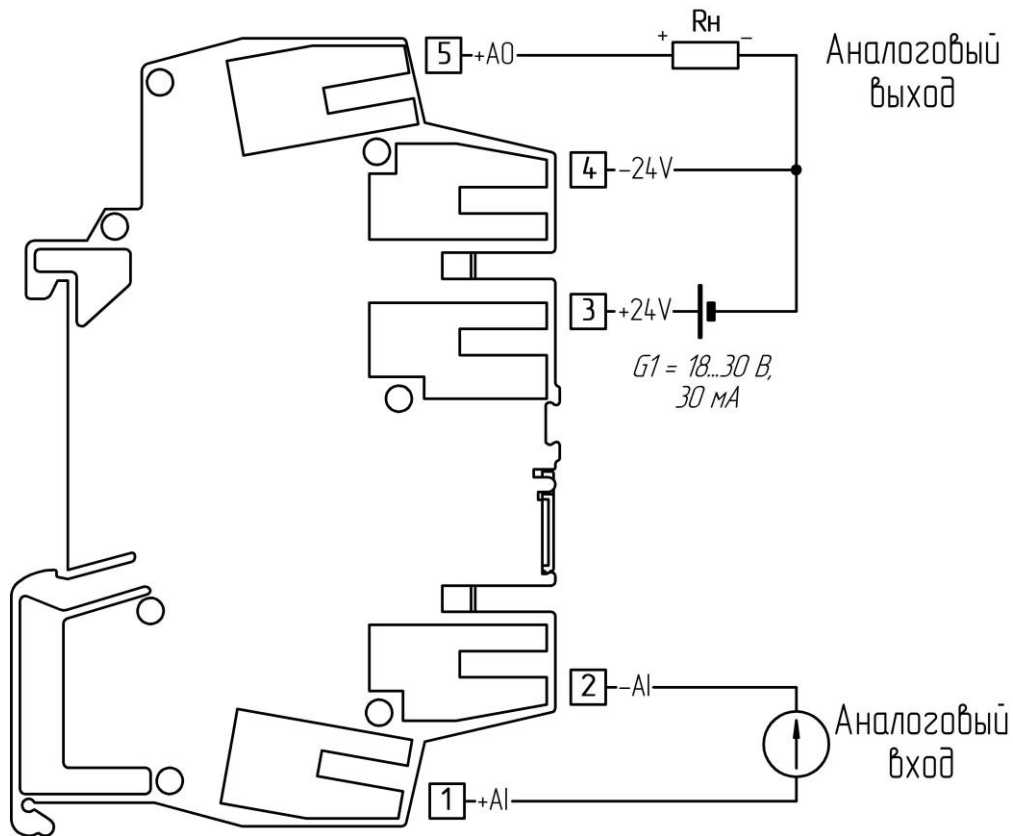
Рисунок 3.4 - Схема внешних соединений преобразователя ПНС-651
