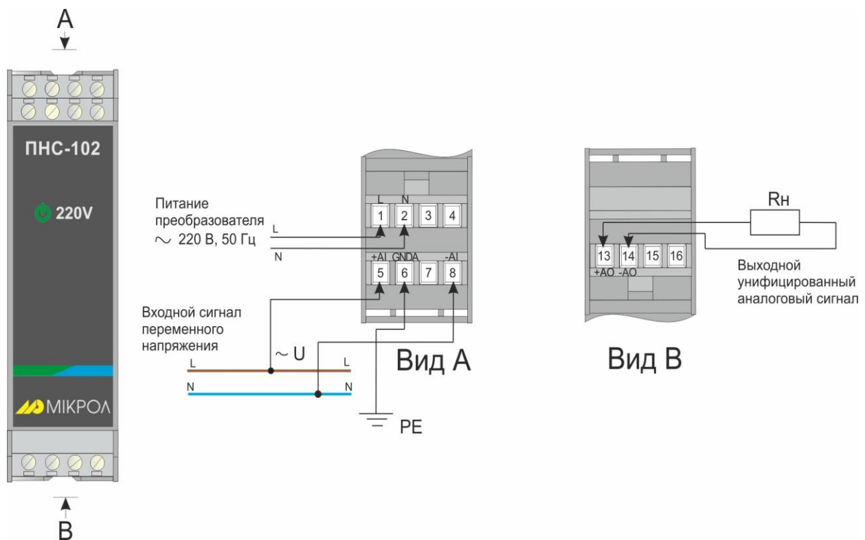
Рисунок 3.4 - Схема электрическая подключений преобразователя ПНС-102
