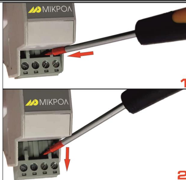
Рисунок 3.3 – Схема извлечения разъем-клеммы с помощью плоской отвертки
