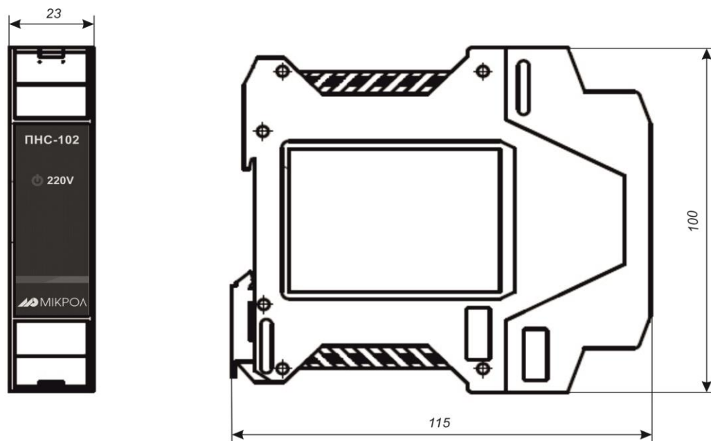
Рисунок 1.1 – Внешний вид и габаритные размеры ПНС-102
