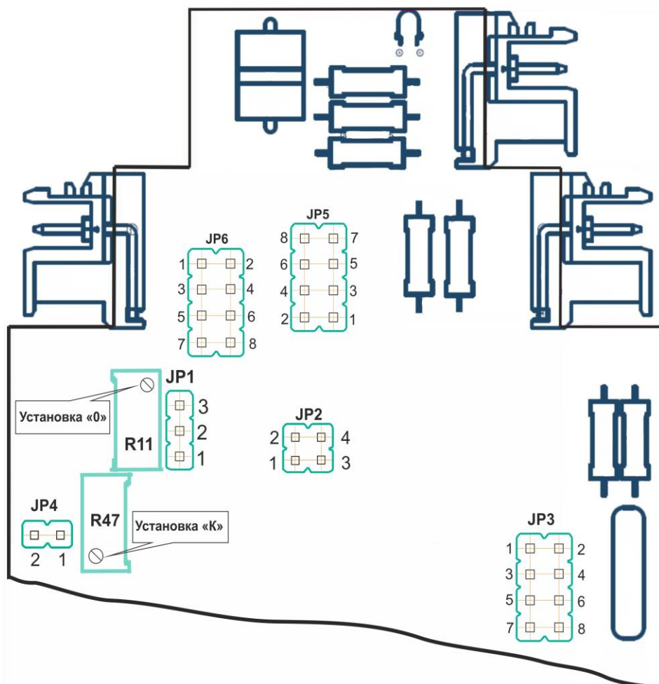
Рисунок 3.1 - Размещение блоков перемычек выбора входных и выходных сигналов
