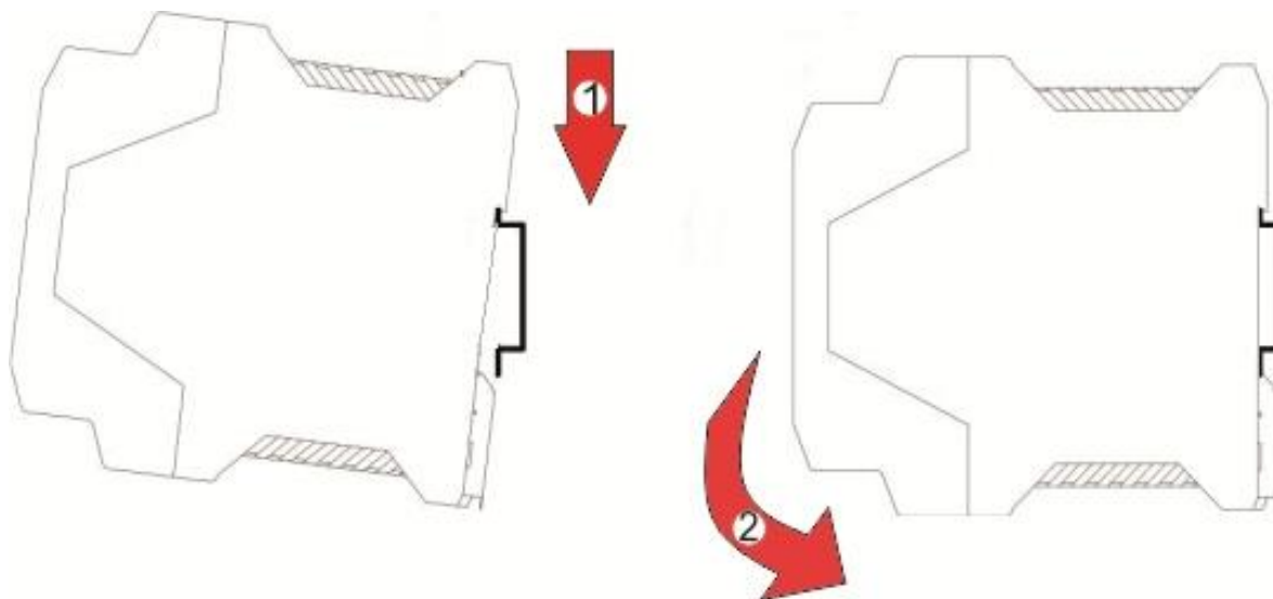
Рисунок 3.2 – Схема крепления преобразователя ПНС-102 на DIN-рельсе
