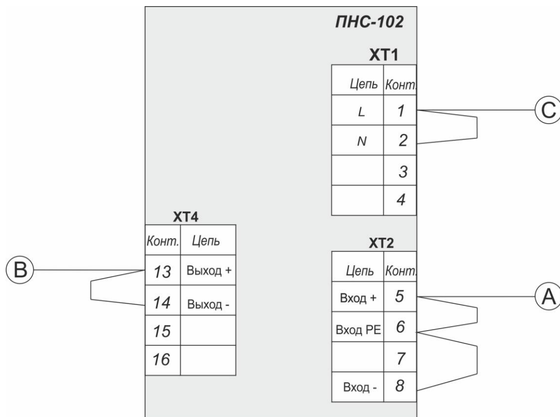
Рисунок Б.1 – Схема проверки сопротивления изоляции
