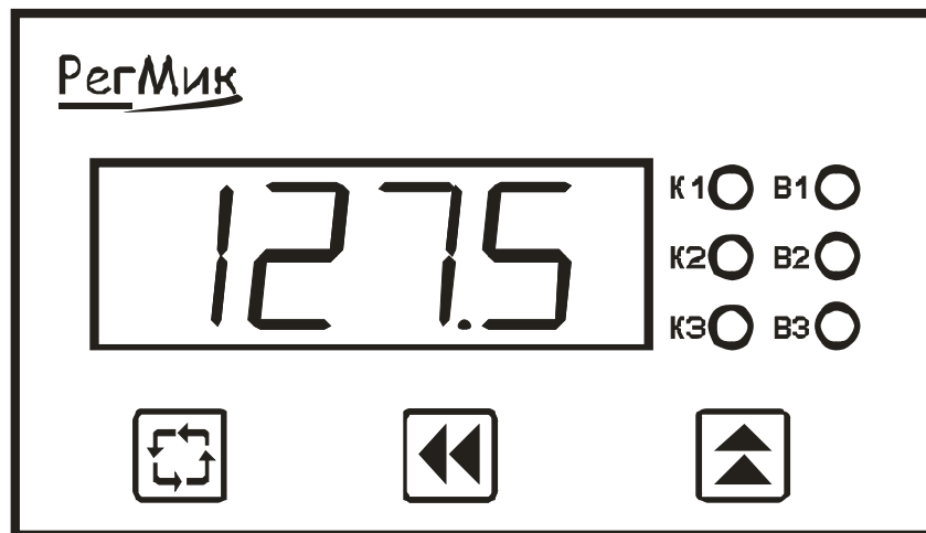
Рисунок 3.2 – Лицевая панель прибора
