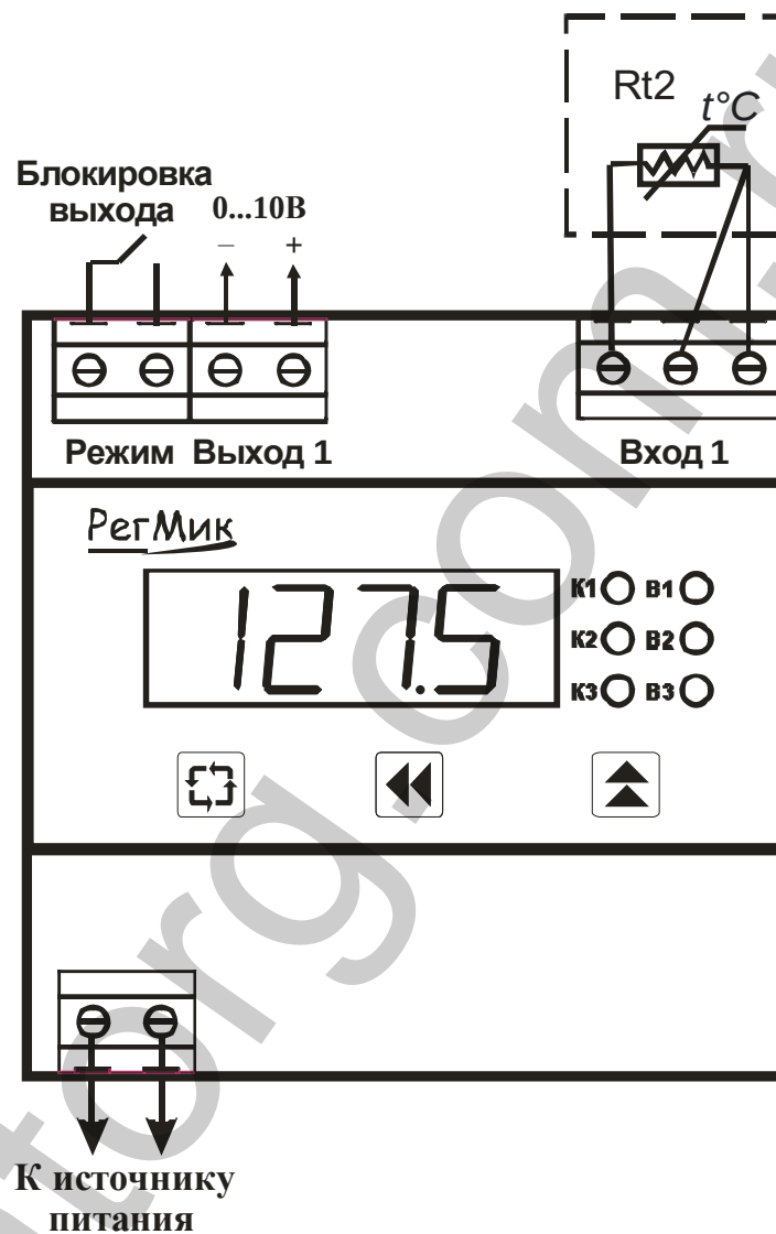
Рисунок 8.1 – Схема подключения ТС, источника питания, исполнительного устройства и интерфейса RS-485
