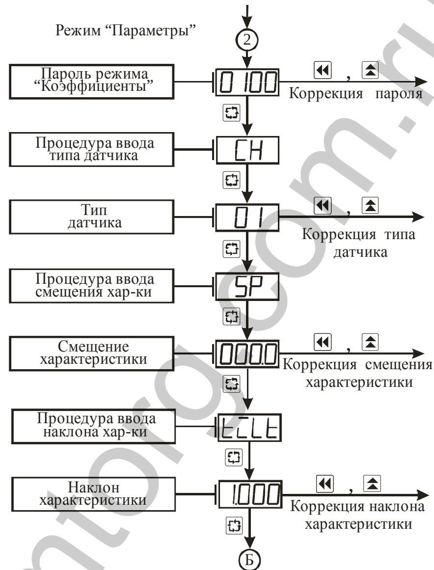
Рисунок 3.4 – Схема алгоритма работы в режиме “Параметры”
