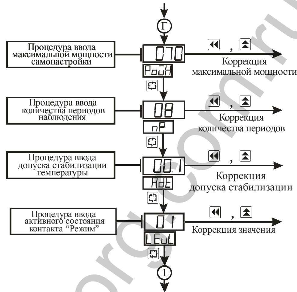
Рисунок 3.12 – Схема алгоритма работы в режиме “Константы ПИД” (окончание)
