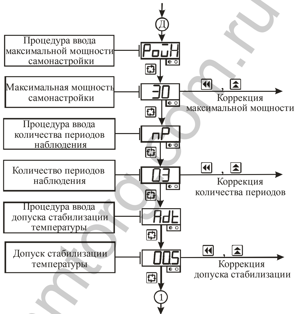
Рисунок 3.13 – Схема алгоритма работы в режиме “Константы ПИД” (окончание)
