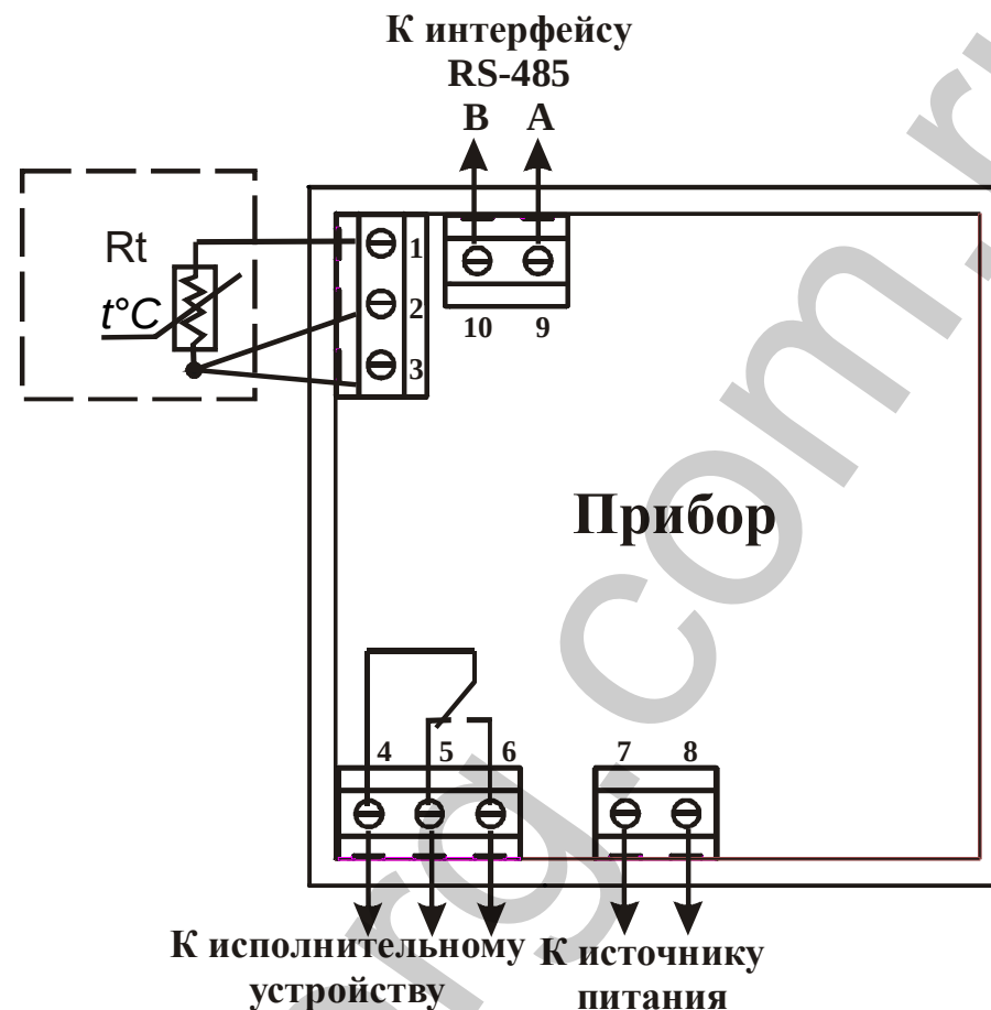
Рисунок 8.1 – Схема подключения ТС, источника питания, исполнительного устройства и интерфейса RS-485
