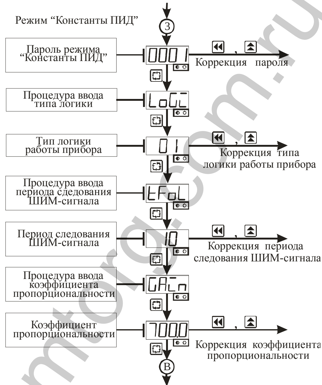
Рисунок 3.10 – Схема алгоритма работы в режиме "Константы ПИД"
