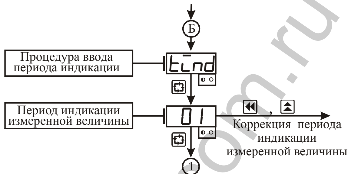
Рисунок 3.6 – Схема алгоритма работы в режиме “Параметры” (окончание)
