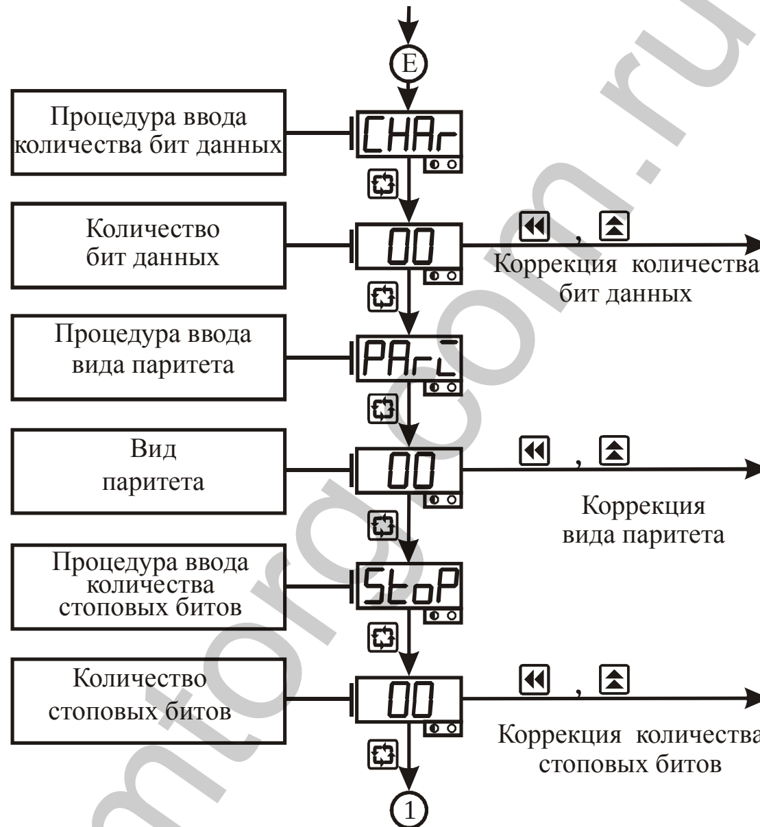
Рисунок 3.17 – Схема алгоритма работы в режиме “Настройка RS-485” (окончание)
