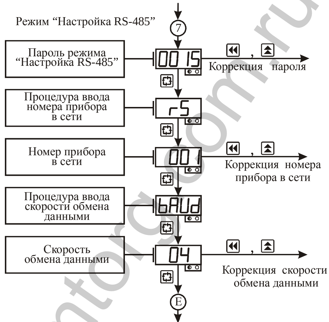
Рисунок 3.16 – Схема алгоритма работы в режиме "Настройка RS-485"
