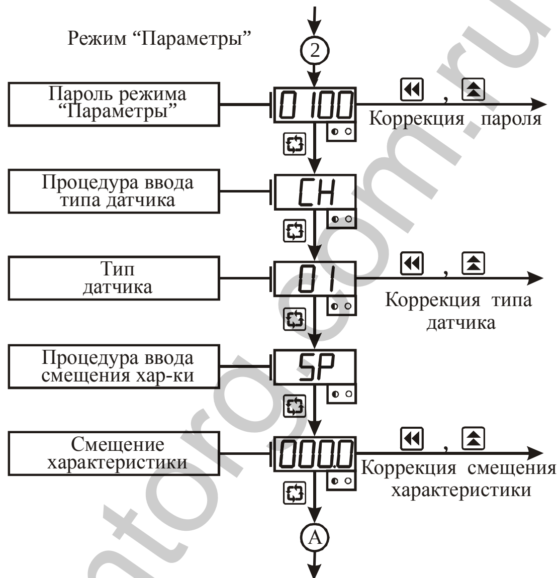
Рисунок 3.4 – Схема алгоритма работы в режиме "Параметры"
