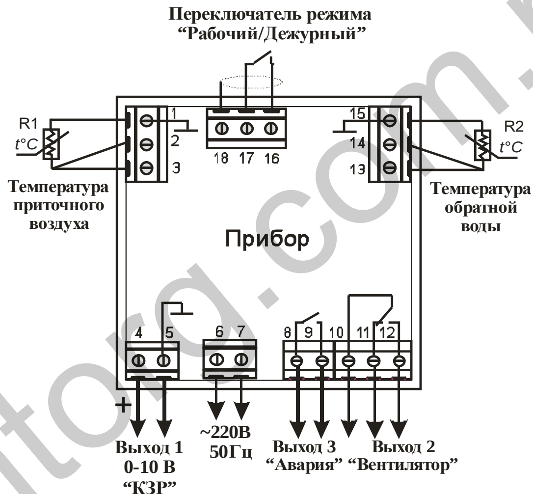
Рисунок 8.1 – Схема подключения ТС, источника питания и исполнительных устройств
