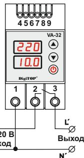
Схема подключения
