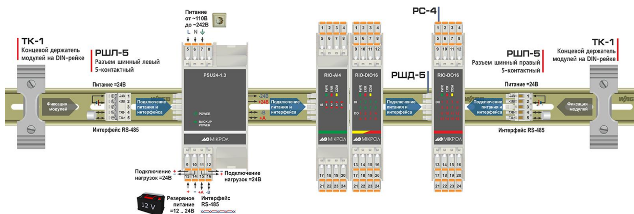
Рисунок Б.3 - Схема внешних соединений RIO-RPM3 с блоком питания и другими модулями
