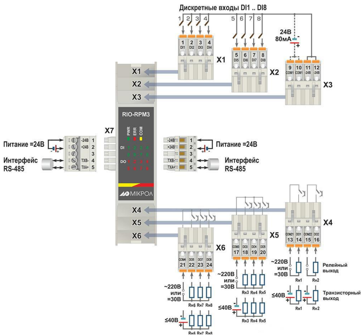
Рисунок Б.1 – Нумерация клемм и сигналы модуля тахометров RIO-RPM3 для исполнения дискретных входов с общим минусом (однополярное исполнение):
