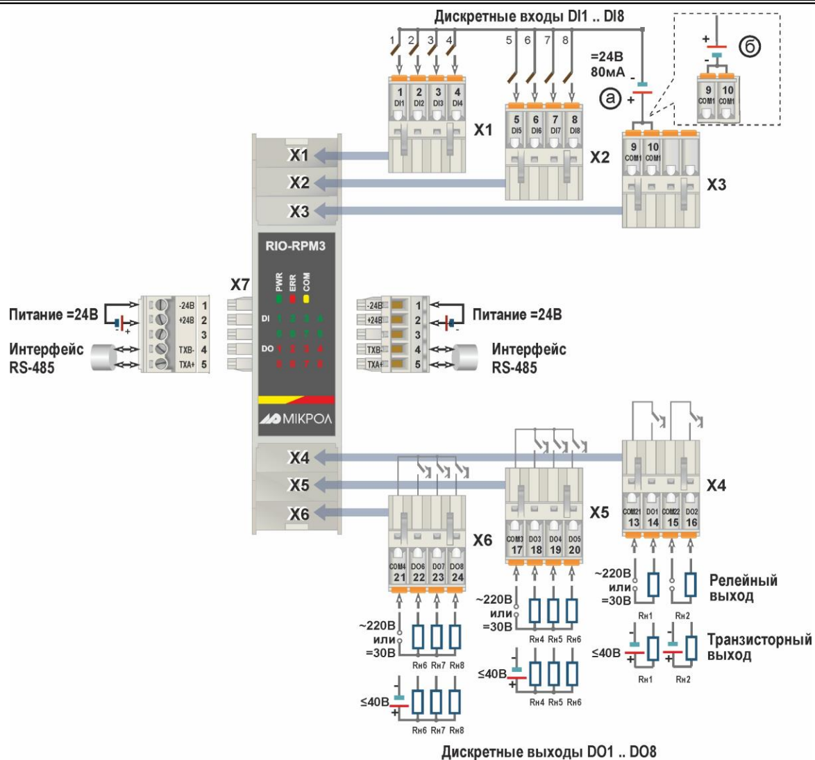
Рисунок Б.2 – Нумерация клемм и сигналы модуля тахометров RIO-RPM3 для исполнения дискретных входов с общим любой полярности (двухполярное исполнение):
