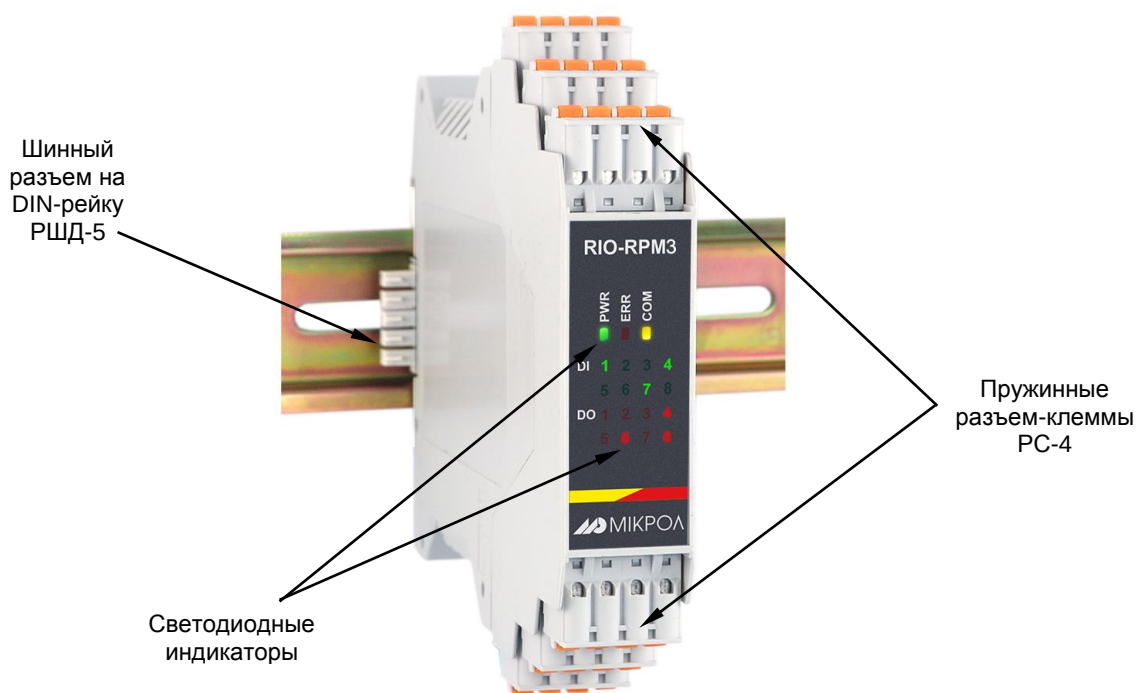
Рисунок. 3.1 - Внешний вид модуля RIO-RPM3
