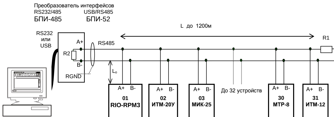
Рисунок Б.4 - Организация интерфейсной связи между ПК и устройствами
