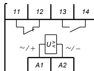
A1, A2 – контролируемое напряжение 11, 12, 13, 14 – контакты для подключения нагрузки
