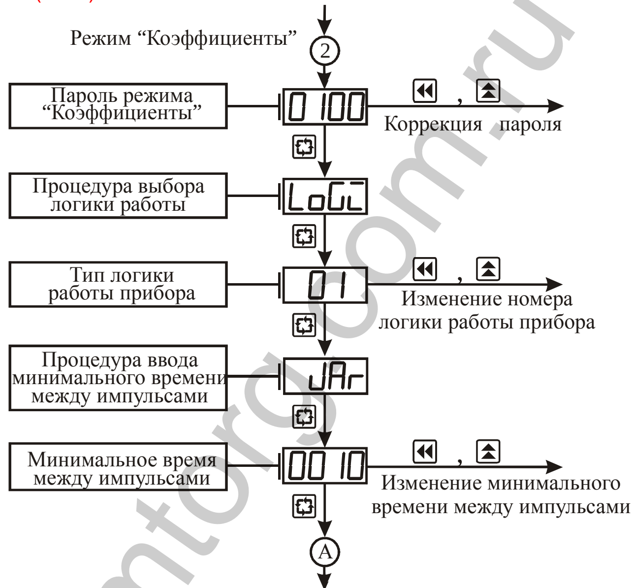
Рисунок 3.4 – Схема алгоритма работы в режиме “Коэффициенты”
