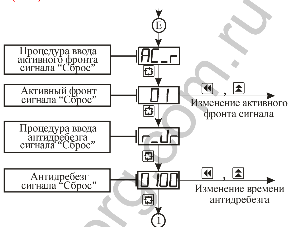
Рисунок 3.10 – Схема алгоритма работы в режиме “Коэффициенты” (окончание)
