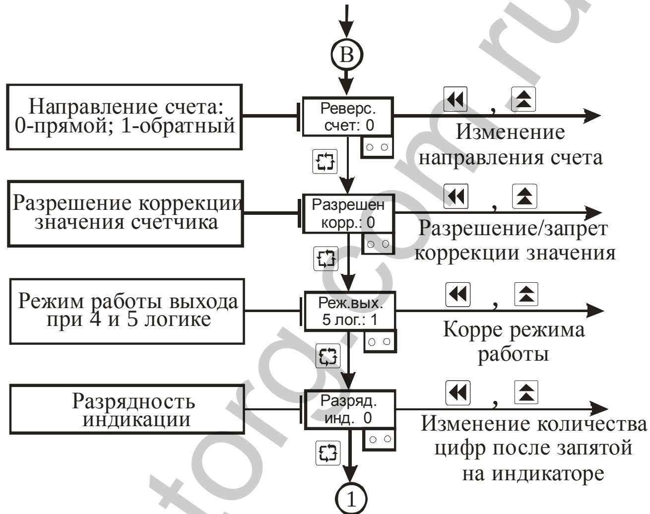
Рисунок 3.9 – Схема алгоритма работы в подрежиме “Коэффициенты 1-го канала” (окончание)
