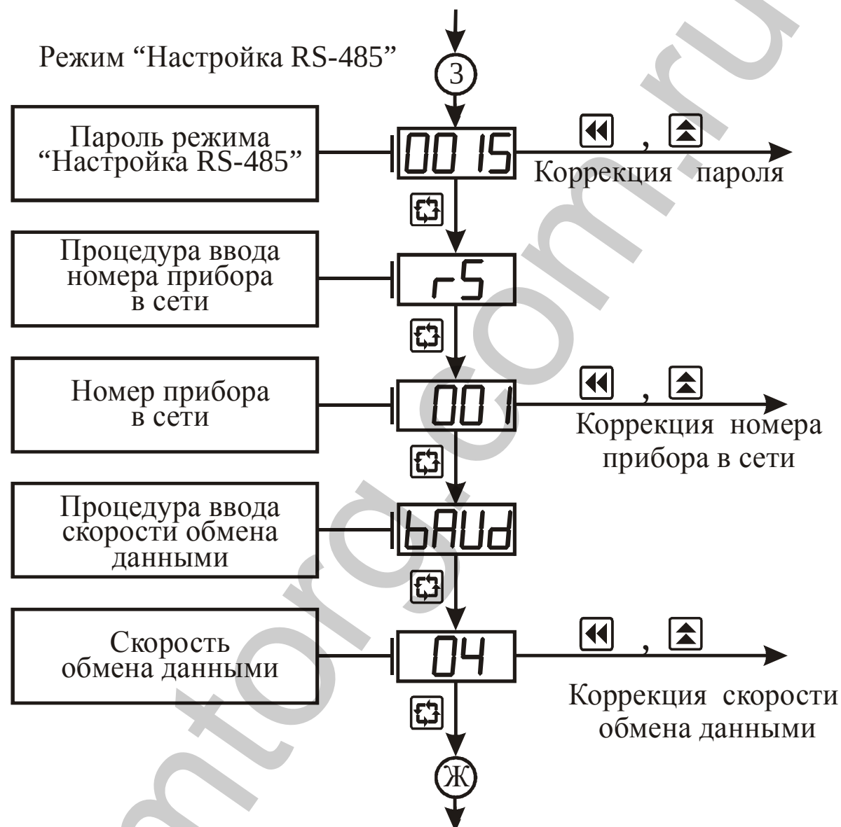
Рисунок 3.11 – Схема алгоритма работы в режиме "Настройка RS-485"
