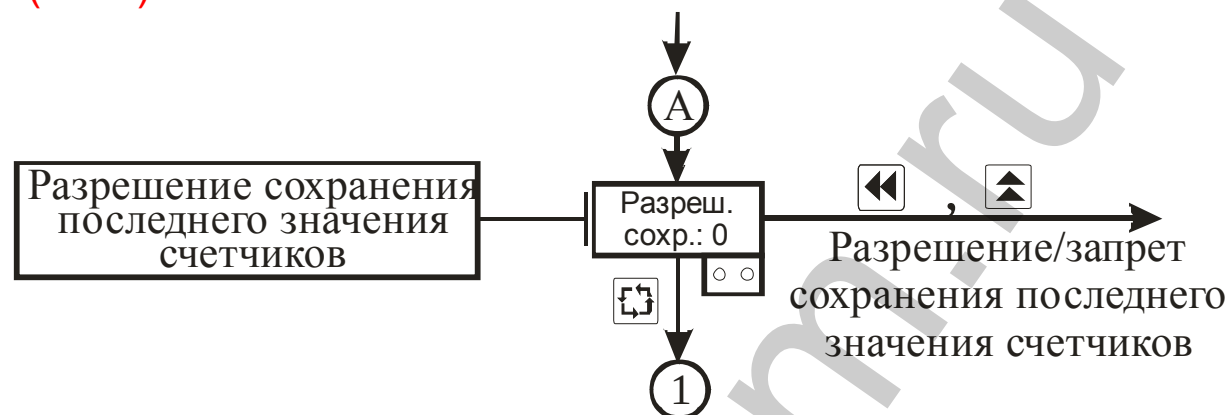
Рисунок 3.6 – Схема алгоритма работы прибора в режиме “Общие параметры” (окончание)
