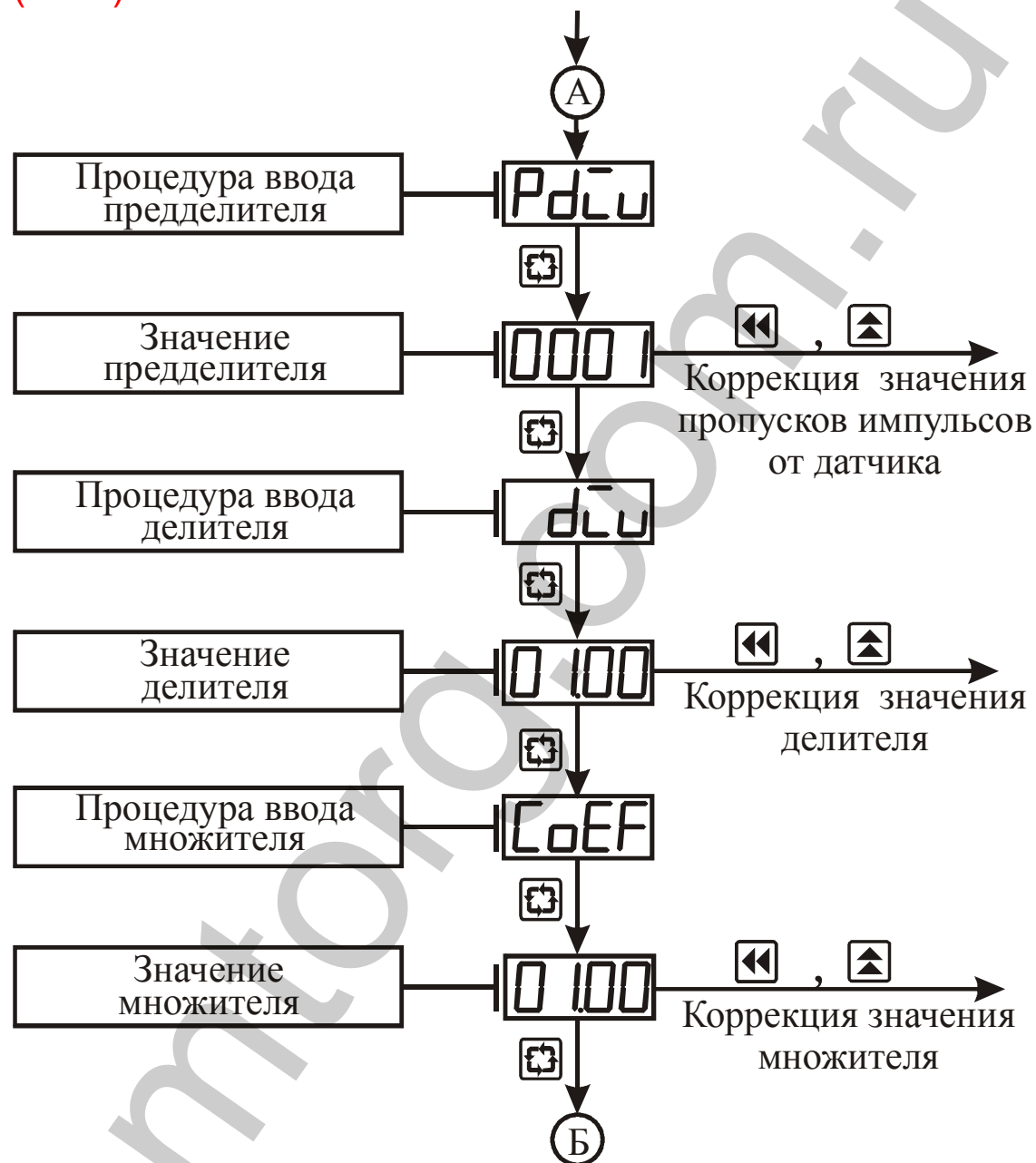
Рисунок 3.5 – Схема алгоритма работы в режиме “Коэффициенты” (продолжение)
