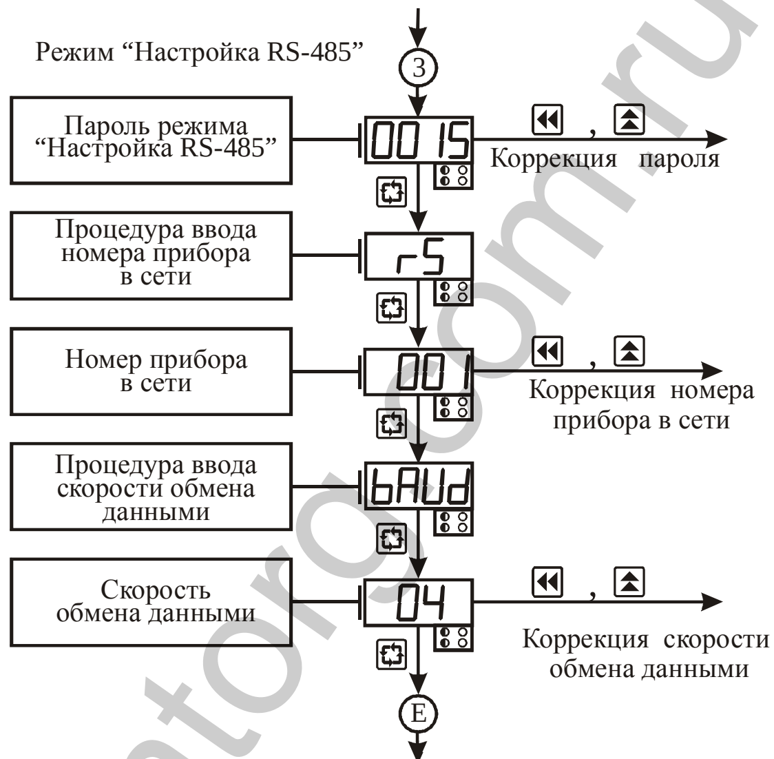
Рисунок 3.10 – Схема алгоритма работы в режиме "Настройка RS-485"
