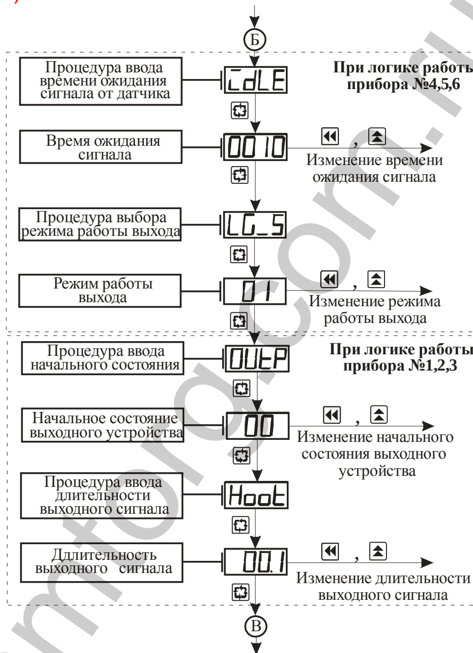
Рисунок 3.6 – Схема алгоритма работы в режиме “Коэффициенты” (продолжение)
