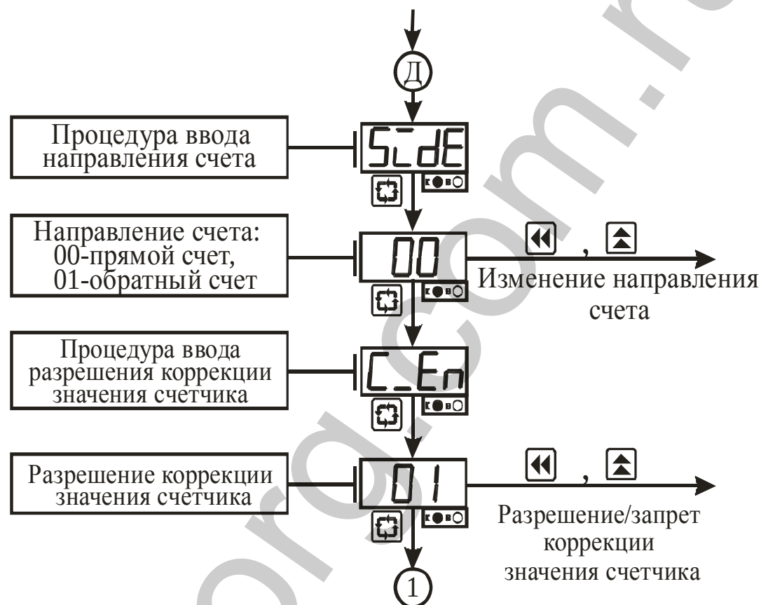
Рисунок 3.9 – Схема алгоритма работы в режиме “Коэффициенты” (окончание)
