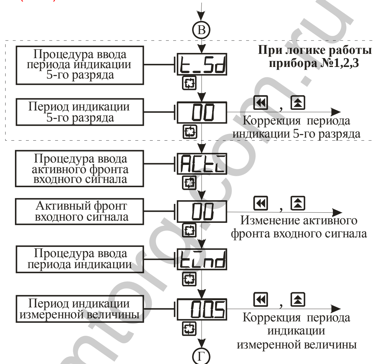
Рисунок 3.7 – Схема алгоритма работы в режиме “Коэффициенты” (продолжение)
