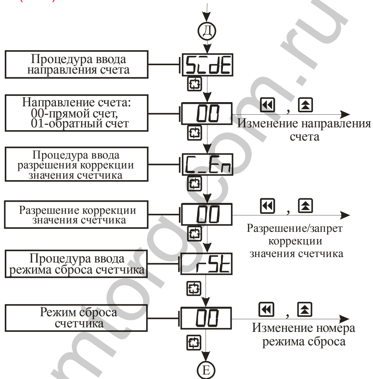
Рисунок 3.9 – Схема алгоритма работы в режиме “Коэффициенты” (продолжение)
