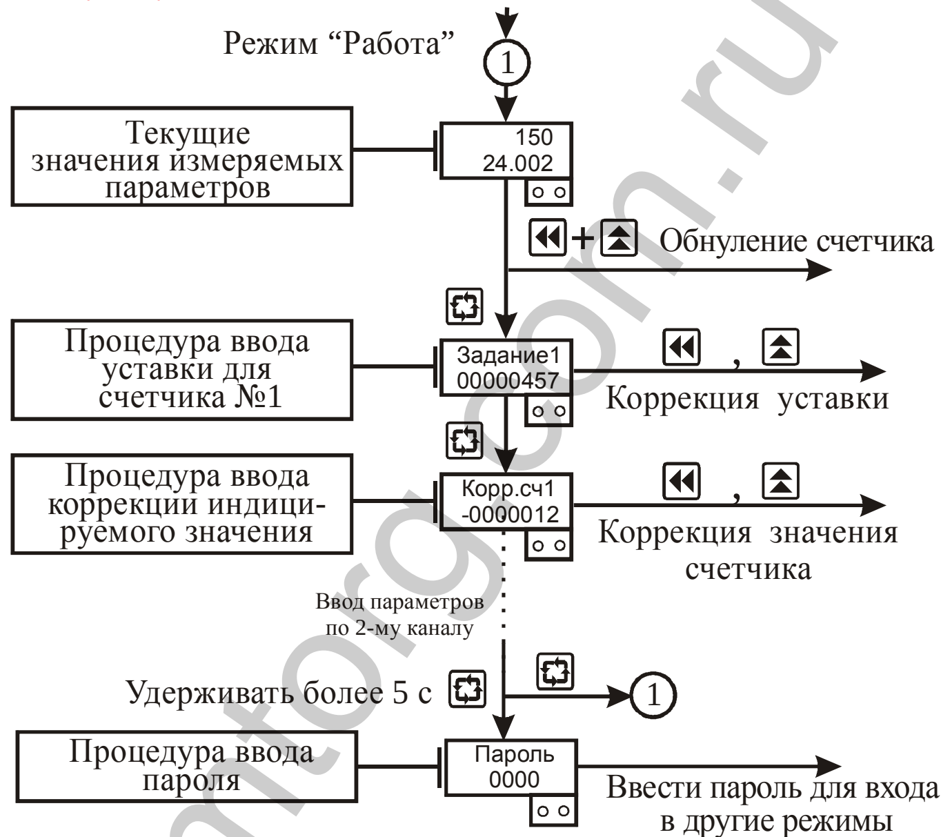
Рисунок 3.3 – Схема алгоритма работы прибора в режиме "Работа"
