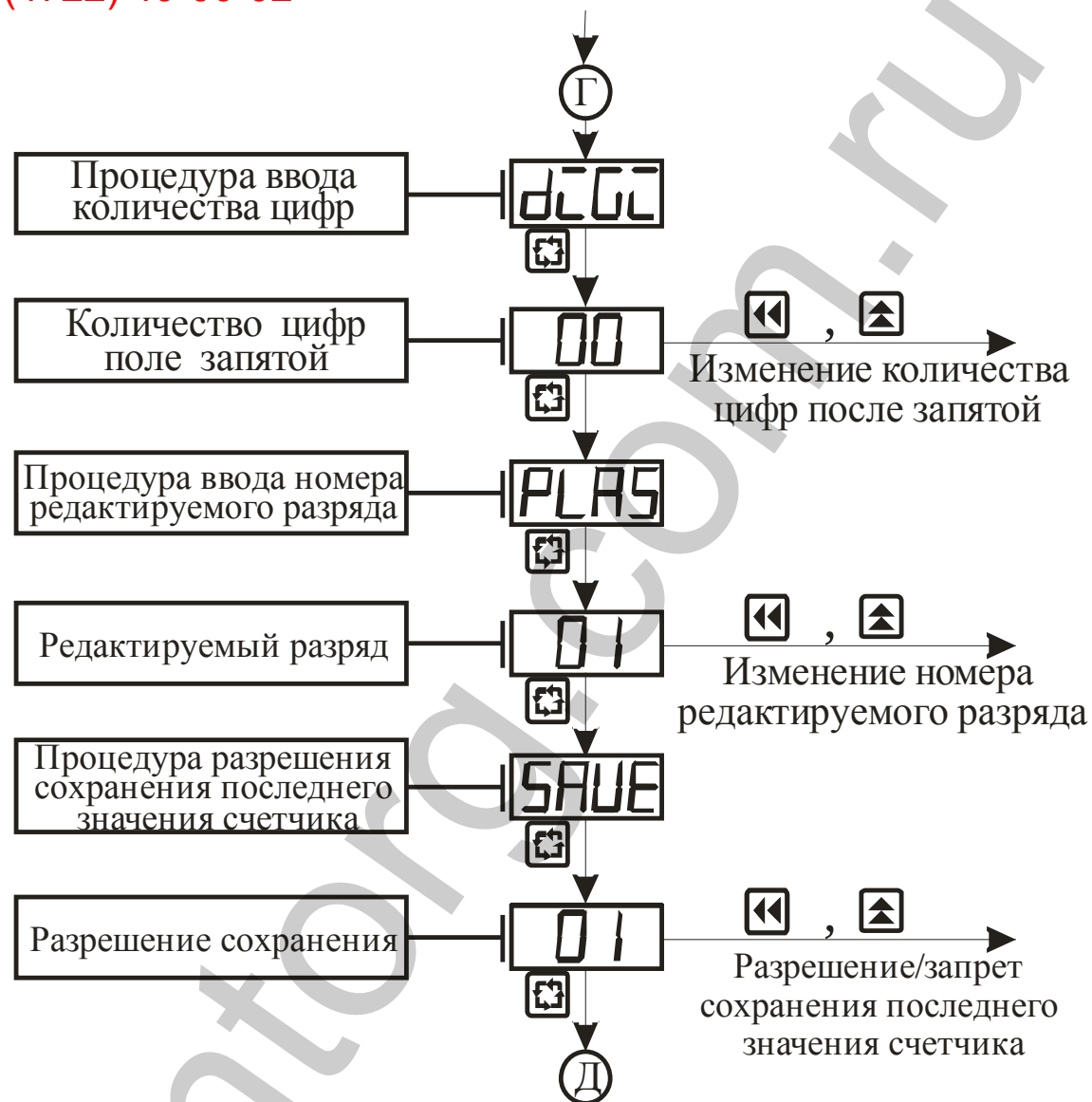
Рисунок 3.8 – Схема алгоритма работы в режиме “Коэффициенты” (продолжение)
