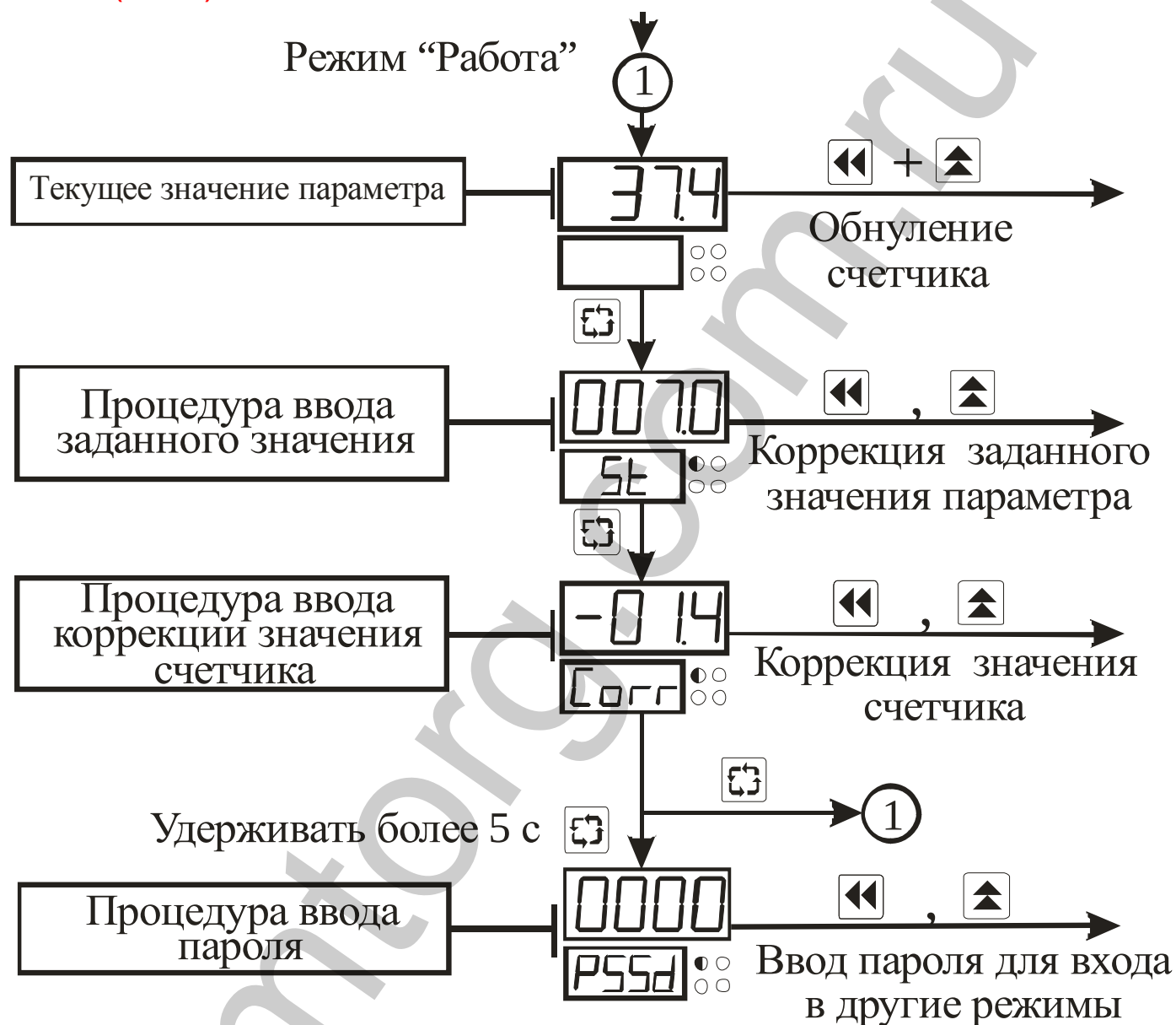
Рисунок 3.3 – Схема алгоритма работы прибора в режиме "Работа"
