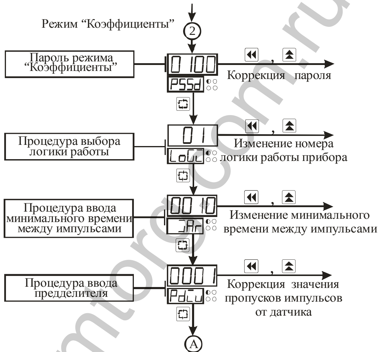
Рисунок 3.3 – Схема алгоритма работы в подрежиме "Коэффициенты 1-го канала"
