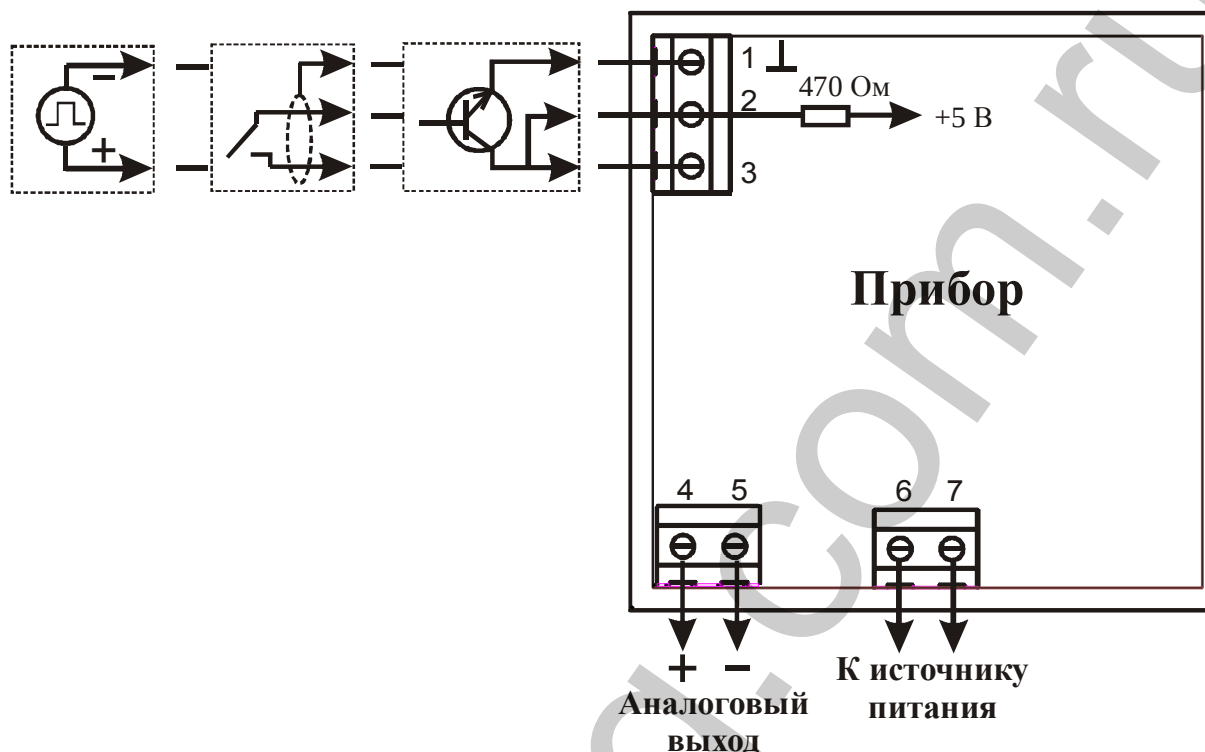
Рисунок 8.1 – Схема подключения входного датчика, источника питания и исполнительных устройств
