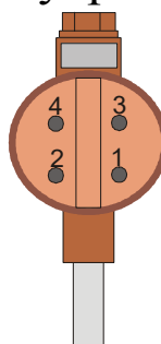
Рисунок 2 – Расположение клемм в контактной колодке
