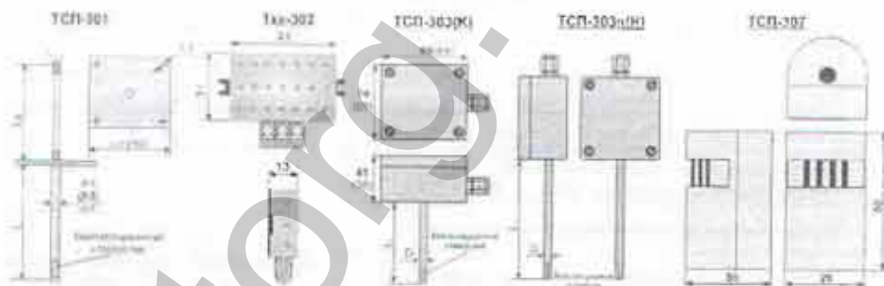
Рисунок 6 - Группа 3. Преобразователи воздушные
