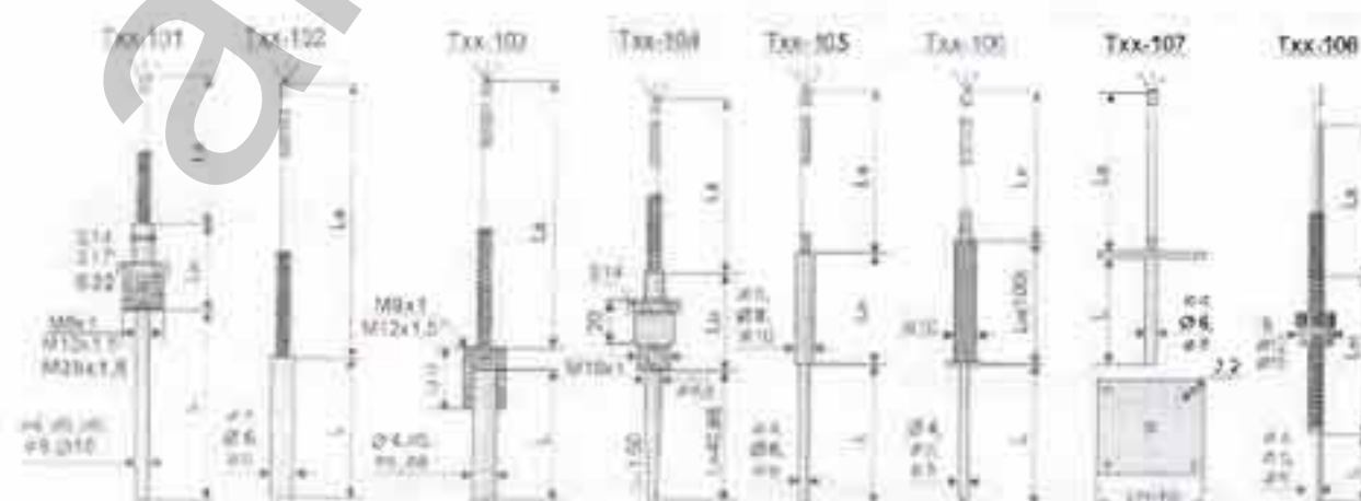
Рисунок 4 - Группа 1. Преобразователи погружаемые с кабельными выводами
