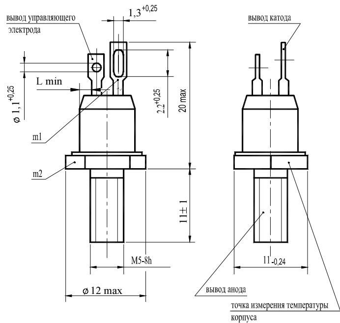
Конструкция тиристоров
