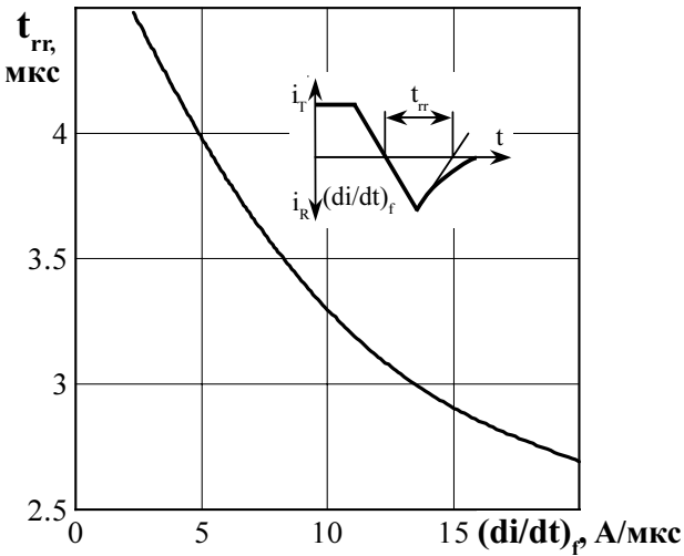
Рисунок 18 - Зависимость времени обратного восстановления t_{rr} от скорости спада тока (di/dt)_r в открытом состоянии при температуре перехода T_{jm} = 125^\circ\text{C} , U_{RM} = 100\text{ В} ; I_T = I_{T(AV)} .
