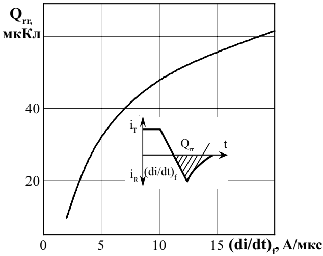
Рисунок 17 - Зависимость заряда восстановления Q_{rr} от скорости спада тока (di/dt)_r в открытом состоянии при температуре перехода T_{jm} = 125^\circ\text{C} , U_{RM} = 100\text{ В} ; I_T = I_{T(AV)} .
