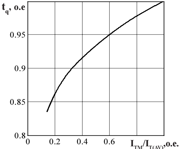
Рисунок 14 - Зависимость времени выключения t_q (о.е.) от амплитуды предшествующего тока в открытом состоянии I_T / I_{T(AV)} (о.е.) при T_{jm} = 125\text{ }^{\circ}\text{C} ; U_R = 100\text{ В} ; (di/dt)_f = 5\text{ А/мкс} ; dU_D/dt = 50\text{ В/мкс} ; U_D = 0,67\text{ } U_{DRM}
