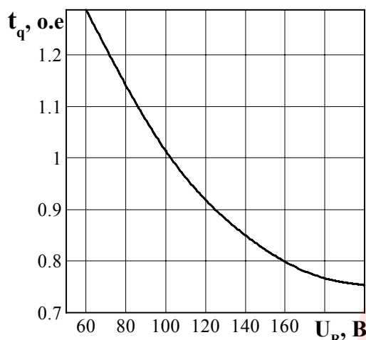
Рисунок 13 - Зависимость времени выключения t_q (о.е.) от обратного напряжения U_R при максимальной температуре перехода T_{im} = 125^\circ \text{C} ; I_T = I_{T(AV)} ; (di/dt)_f = 5 \text{ А/мкс} ; dU_D/dt = 50 \text{ В/мкс} ; U_D = 0,67 U_{DRM}
