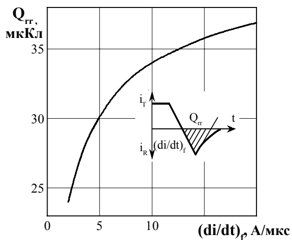
Рисунок 17 - Зависимость заряда восстановления Q_{гр} от скорости спада тока (di/dt)_р в открытом состоянии при температуре перехода T_{jm} = 125^\circ\text{C} , U_{RM} = 100\text{ В} ; I_T = I_{T(AV)} .
