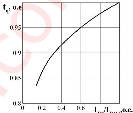
Рисунок 14 - Зависимость времени выключения t_q (о.е.) от амплитуды предшествующего тока в открытом состоянии I_{TM} / I_{T(AV)} (о.е.) при T_{im} = 125^\circ \text{C} ; U_R = 100 \text{ В} ; (di/dt)_f = 5 \text{ А/мкс} ; dU_D/dt = 50 \text{ В/мкс} ; U_D = 0,67 U_{DRM}
