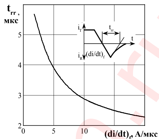
Рисунок 18 - Зависимость времени обратного восстановления t_{гр} от скорости спада тока (di/dt)_р в открытом состоянии при температуре перехода T_{jm} = 125^\circ\text{C} , U_{RM} = 100\text{ В} ; I_T = I_{T(AV)} .
