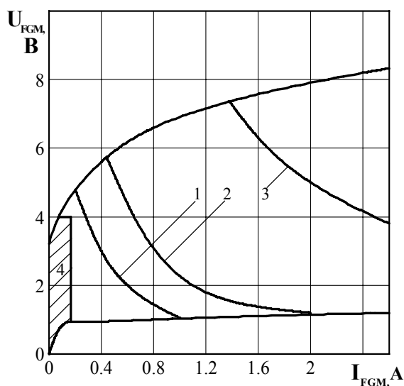
Рисунок 12 - Пределные характеристики цепи управления
