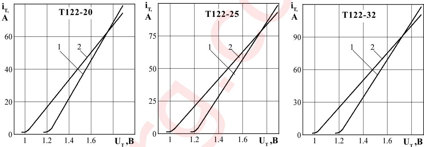
Рисунок 1 - Пределная вольтамперная характеристика в открытом состоянии при температуре перехода 25 °C (1) и максимальной температуре перехода T jm (2) I T = 3,14I T(AV)
