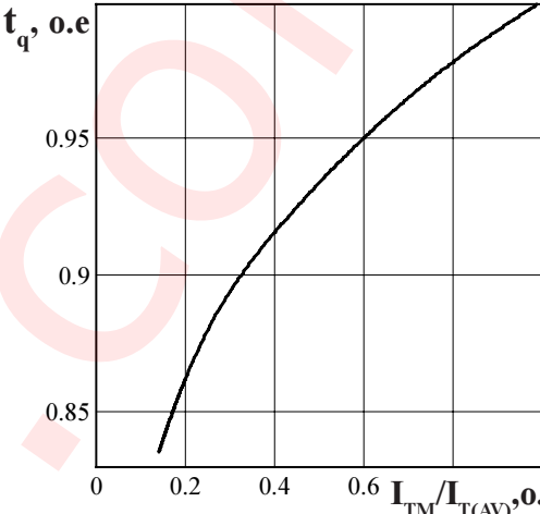
Рисунок 14 - Зависимость времени выключения t_q (о.е.) от амплитуды предшествующего тока в открытом состоянии I_T / I_{T(AV)} (о.е.) при T_{jm} = 125\text{ }^{\circ}\text{C} ; U_R = 100\text{ В} ; (di/dt)_f = 5\text{ А/мкс} ; dU_D/dt = 50\text{ В/мкс} ; U_D = 0,67\text{ }U_{DRM}
