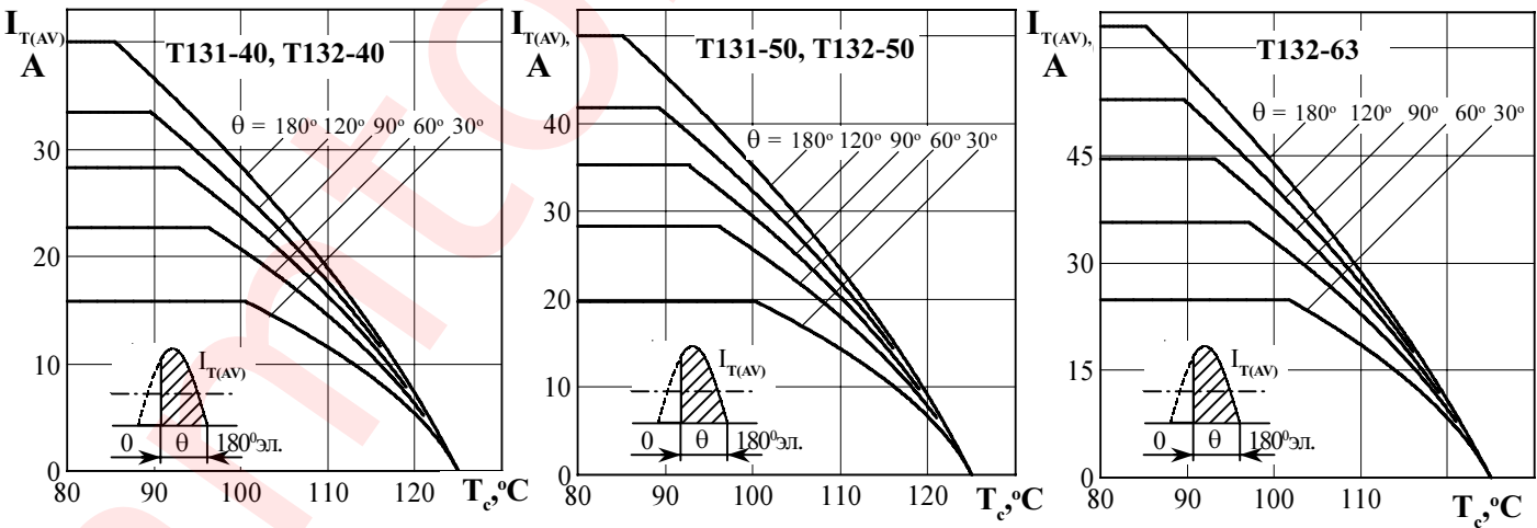
Рисунок 2 - Зависимость допустимого среднего тока в открытом состоянии I T(AV) от температуры корпуса T с для токов синусоидальной формы частотой f = 50 Гц
