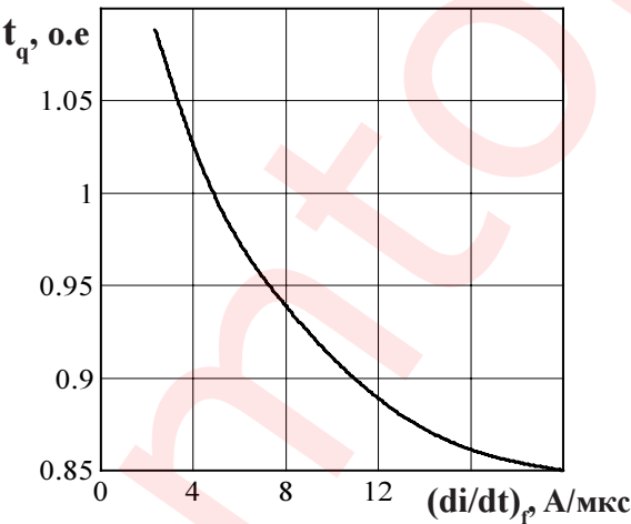
Рисунок 15 - Зависимость времени выключения t_q (о.е.) от скорости спада тока в открытом состоянии (di/dt)_f при T_{jm} = 125\text{ }^{\circ}\text{C} ; I_T = I_{T(AV)} ; U_R = 100\text{ В} ; dU_D/dt = 50\text{ В/мкс} ; U_D = 0,67\text{ }U_{DRM}
