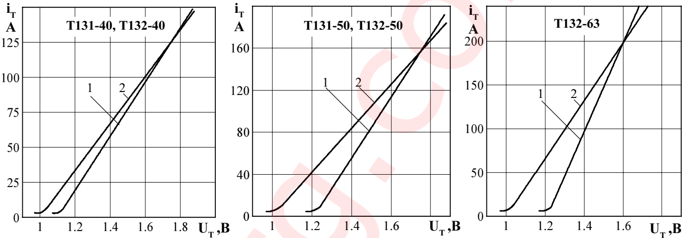
Рисунок 1 - Предельная вольтамперная характеристика в открытом состоянии при температуре перехода 25 °С (1) и максимальной температуре перехода T жм (2) I T = 3,14I T(AV)
