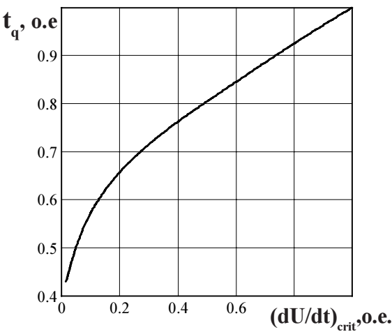
Рисунок 16 - Зависимость времени выключения t_q (о.е.) от скорости нарастания напряжения в закрытом состоянии dU_D/dt при T_{jm} = 125\text{ }^{\circ}\text{C} ; I_T = I_{T(AV)} ; U_D = 0,67\text{ }U_{DRM} ; U_R = 100\text{ В} ; (di/dt)_f = 5\text{ А/мкс}
