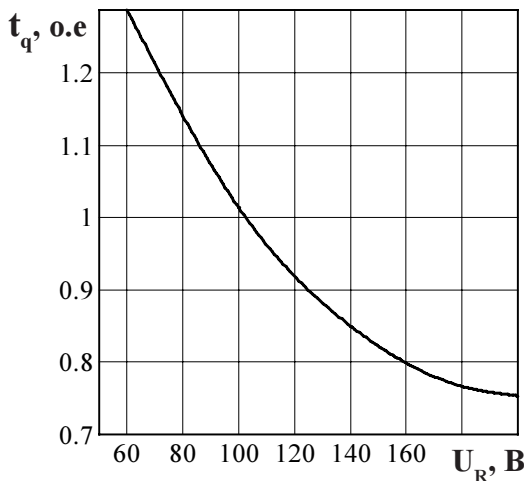
Рисунок 13 - Зависимость времени выключения t_q (о.е.) от обратного напряжения U_R при максимальной температуре перехода T_{jm} = 125^\circ \text{C} ; I_T = I_{T(AV)} ; (di/dt)_f = 5 \text{ А/мкс} ; dU_D/dt = 50 \text{ В/мкс} ; U_D = 0,67 U_{DRM}
