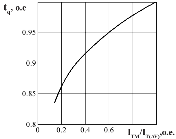
Рисунок 14 - Зависимость времени выключения t_q (о.е.) от амплитуды предшествующего тока в открытом состоянии I_T / I_{T(AV)} (о.е.) при T_{jm} = 125^\circ \text{C} ; U_R = 100 \text{ В} ; (di/dt)_f = 5 \text{ А/мкс} ; dU_D/dt = 50 \text{ В/мкс} ; U_D = 0,67 U_{DRM}
