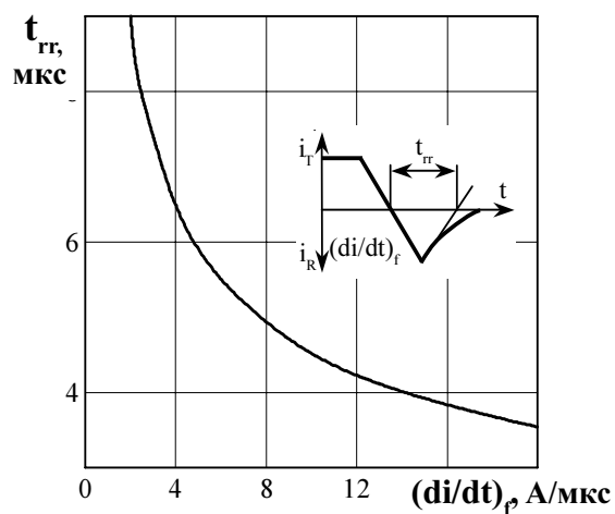
Рисунок 18 - Зависимость времени обратного восстановления t_{rr} от скорости спада тока (di/dt)_f в открытом состоянии при температуре перехода T_{jm} = 125^\circ\text{C} , U_{RM} = 100\text{ В} ; I_T = I_{T(AV)} .
