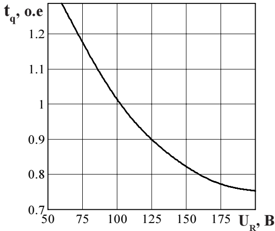
Рисунок 13 - Зависимость времени выключения t_q (о.е.) от обратного напряжения U_R при максимальной температуре перехода T_{im} = 125\text{ }^{\circ}\text{C} ; I_T = I_{T(AV)} ; (di/dt)_f = 5\text{ А/мкс} ; dU_D/dt = 50\text{ В/мкс} ; U_D = 0,67 U_{DRM}
