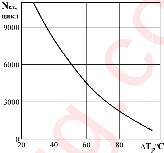
Рисунок 19 - Зависимость максимально допустимого числа циклов N_{ст.} от перепада температуры перехода \Delta T_j при циклической токовой нагрузке.
