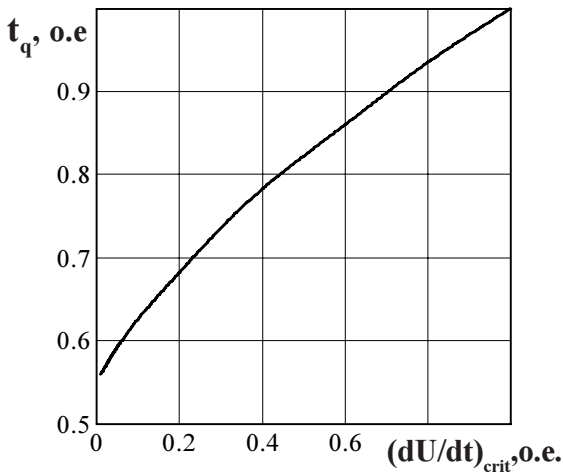
Рисунок 16 - Зависимость времени выключения t_q (о.е.) от скорости нарастания напряжения в закрытом состоянии dU_D/dt при T_{im} = 125\text{ }^{\circ}\text{C} ; I_T = I_{T(AV)} ; U_D = 0,67 U_{DRM} ; U_R = 100\text{ В} ; (di/dt)_f = 5\text{ А/мкс}
