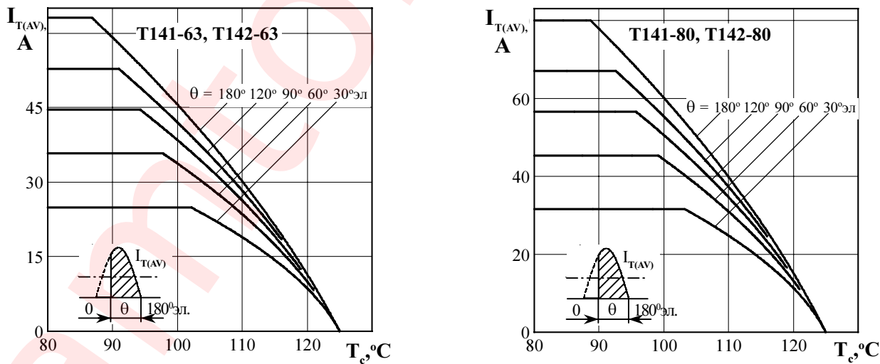
Рисунок 2 - Зависимость допустимого среднего тока в открытом состоянии I T(AV) от температуры корпуса T c для токов синусоидальной формы частотой f = 50 Гц
