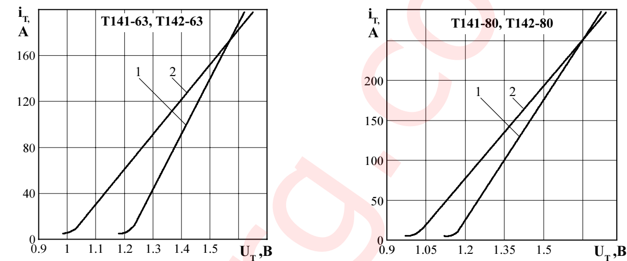
Рисунок 1 - Предельная вольт-амперная характеристика в открытом состоянии при температуре перехода 25 °C (1) и максимальной температуре перехода T jm (2) I T = 3,14I T(AV)
