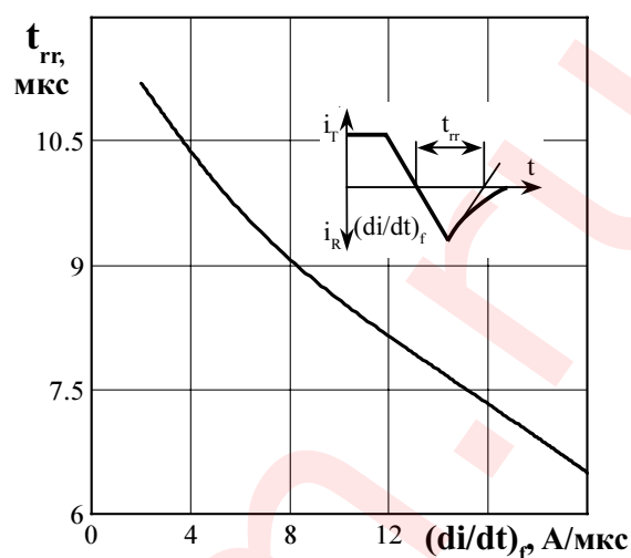
Рисунок 18 - Зависимость времени обратного восстановления t_{rr} от скорости спада тока (di/dt)_f в открытом состоянии при температуре перехода T_{jm} = 125^\circ\text{C} , U_{RM} = 100\text{ В} ; I_T = I_{T(AV)} .
