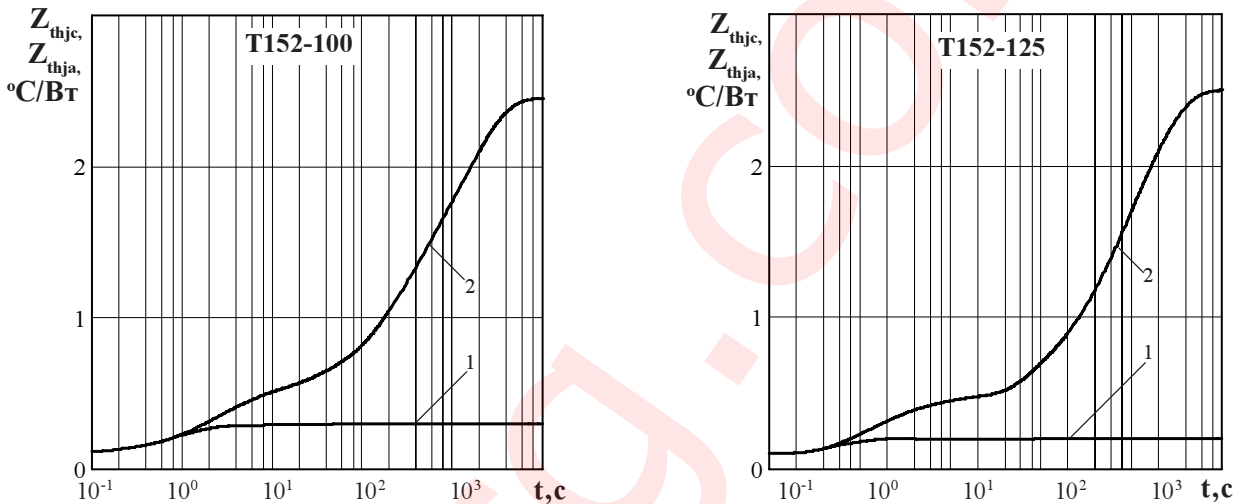
Рисунок 11 - Зависимость теплового сопротивления переход - корпус Z_{thjc} (1) и переход- среда Z_{thja} (2) от времени t при естественном охлаждении T_a = 40^\circ\text{C} на типовом охладителе
