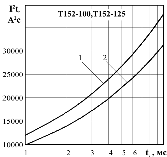
Рисунок 9 - Зависимость защитного показателя I^2t от длительности импульса тока t_i при исходной температуре структуры T_j = 25^\circ\text{C} (1) и максимальной температуре T_{jm} (2)
