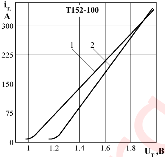
Рисунок 1 - Пределная вольтамперная характеристика в открытом состоянии при температуре перехода 25 °C (1) и максимальной температуре перехода T jm (2) I T = 3,14I T(AV)
