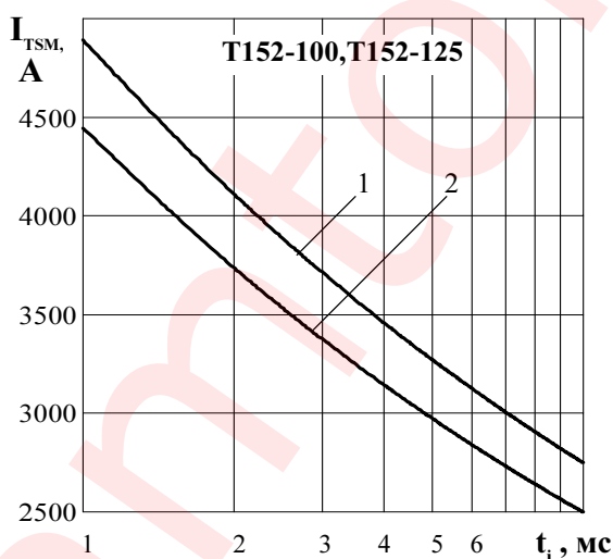
Рисунок 8 - Зависимость допустимой амплитуды ударного тока в открытом состоянии I_{TSM} от длительности импульса тока t_i при исходной температуре структуры T_j = 25^\circ\text{C} (1) и максимальной температуре T_{jm} (2)
