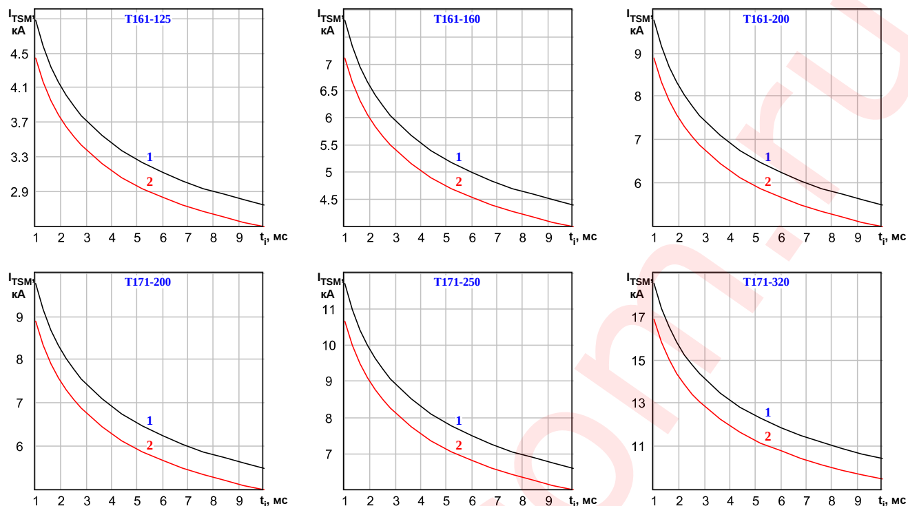
Рисунок 4: Зависимость допустимой амплитуды ударного тока в открытом состоянии I_{TSM} от длительности импульса тока t_i при исходной температуре структуры T_j=25\text{ }^{\circ}\text{C} (1) и максимально допустимой температуре перехода T_{jm} (2).
