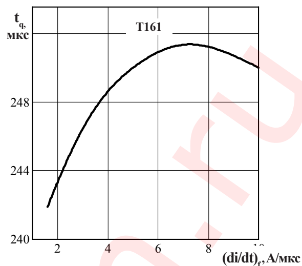
Рисунок 17 - Зависимость времени выключения t_q от скорости спада тока в открытом состоянии (di/dt)_f при T_{jm} = 125^\circ\text{C} ; I_T = I_{T(AV)} ; U_R = 100 \text{ В} ; dU_D/dt = 50 \text{ В/мкс} ; U_D = 0,67 U_{DRM}
