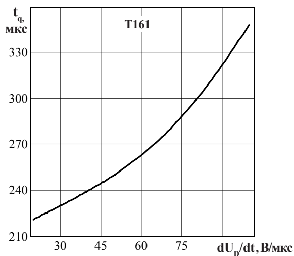
Рисунок 16 - Зависимость времени выключения t_q от скорости нарастания напряжения в закрытом состоянии dU_D/dt при T_{jm} = 125^\circ\text{C} ; I_T = I_{T(AV)} ; U_D = 0,67 U_{DRM} ; U_R = 100 \text{ В} ; (di/dt)_f = 5 \text{ А/мкс}
