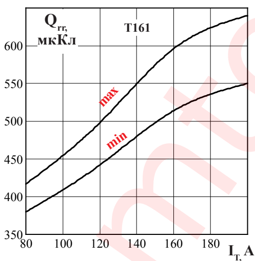
Рисунок 13 - Зависимость заряда восстановления Q_{rr} от амплитуды тока в открытом состоянии I_T при U_R = 100\text{ В} ; T_{jm} = 125^\circ\text{C} ; (di/dt)_f = 5\text{ А/мкс}
