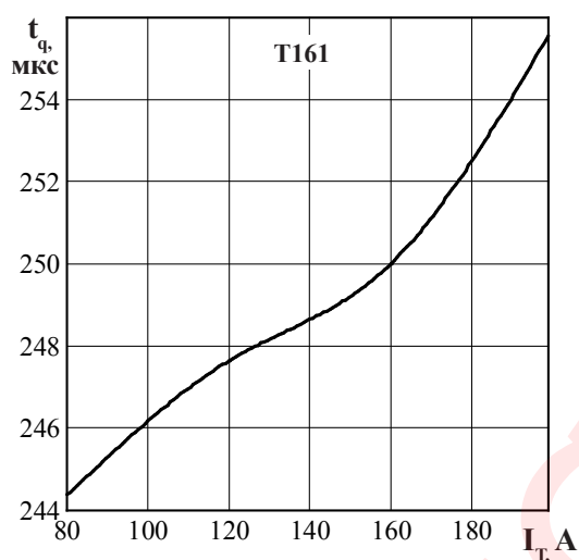
Рисунок 18 - Зависимость времени выключения t_q от амплитуды тока в открытом состоянии I_T при T_{jm} = 125^\circ\text{C} ; U_R = 100 \text{ В} ; (di/dt)_f = 5 \text{ А/мкс} ; dU_D/dt = 50 \text{ В/мкс}
