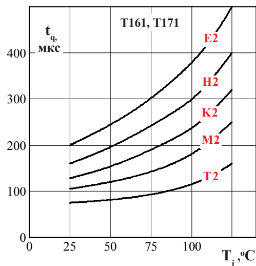
Рисунок 15 - Зависимость времени выключения t_q от температуры структуры T_j при I_T = I_{TAVM} ; U_D = 0,67 U_{DRM} ; U_R = 100\text{ В} ; (di/dt)_f = 5\text{ А/мкс} ; dU_D/dt = 50\text{ В/мкс}
