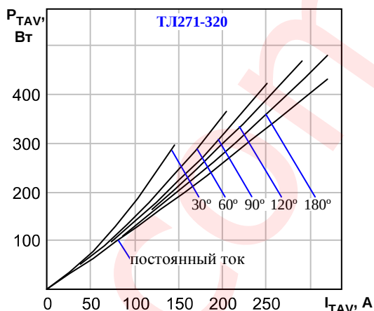
Рисунок 7: Зависимость средней рассеиваемой мощности в открытом состоянии P_{TAV} от среднего тока в открытом состоянии I_{TAV} прямоугольной формы частотой 50 Гц при различных углах проводимости и постоянного тока.
