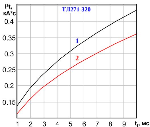
Рисунок 5: Зависимость защитного показателя I^2t от длительности импульса тока t_i при исходной температуре структуры T_j=25\text{ °C} (1) и максимально допустимой температуре перехода T_{jm} (2).
