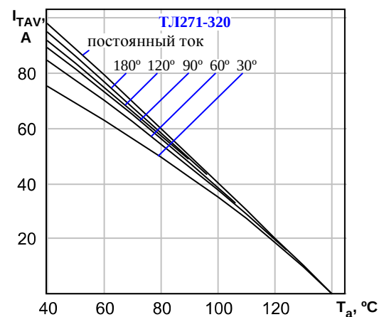
Рисунок 9: Зависимость допустимого среднего тока в открытом состоянии I_{TAV} прямоугольной формы частотой 50 Гц при различных углах проводимости и постоянного тока от температуры окружающей среды T_a при естественном охлаждении на ОР281-110.
