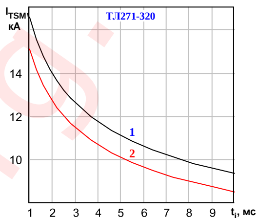
Рисунок 4: Зависимость допустимой амплитуды ударного тока в открытом состоянии I_{TSM} от длительности импульса тока t_i при исходной температуре структуры T_j=25\text{ °C} (1) и максимально допустимой температуре перехода T_{jm} (2).
