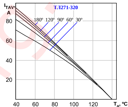
Рисунок 8: Зависимость допустимого среднего тока в открытом состоянии I_{TAV} синусоидальной формы частотой 50 Гц при различных углах проводимости от температуры окружающей среды T_a при естественном охлаждении на ОР281-110.
