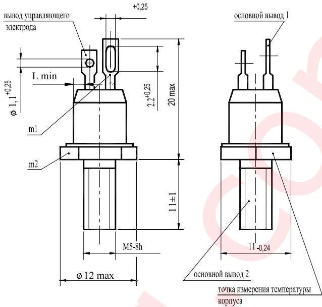
Конструкция триаков
