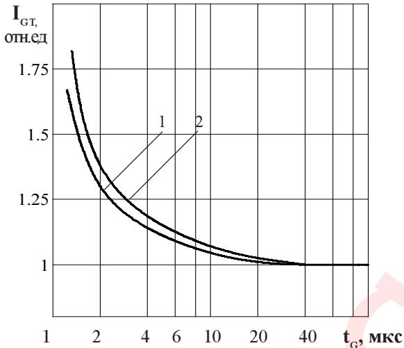
Рисунок 10 - Зависимость отпирающего импульсного тока управления I ГТ от длительности управляющего импульса t Г при температуре перехода T Г = 25 °С (1), T Гmin = минус 50 °С (2) и напряжения в закрытом состоянии U Д = 12 В.
