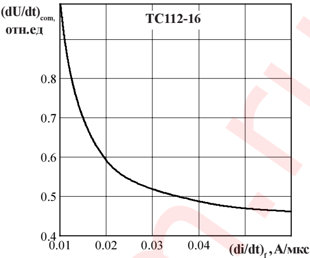
Рисунок 14 - Зависимость критической величины скорости нарастания коммутационного напряжения (dU/dt)_{com} от скорости спада предшествующего тока в открытом состоянии (di_f/dt)_f при амплитуде предшествующего тока в открытом состоянии I_T = I_{TRSM} и максимально допустимой температуре перехода T_{jm} .
