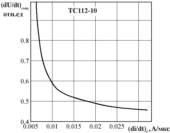
Рисунок 14 - Зависимость критической величины скорости нарастания коммутационного напряжения (dU/dt)_{com} от скорости спада предшествующего тока в открытом состоянии (di_f/dt)_f при амплитуде предшествующего тока в открытом состоянии I_T = I_{TRSM} и максимально допустимой температуре перехода T_{jm} .
