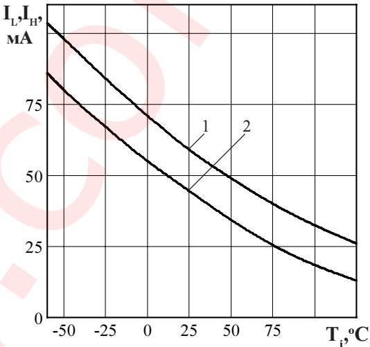
Рисунок 11 - Зависимость тока удержания I Н (1) и тока включения I Л (2) от температуры перехода T Г .
