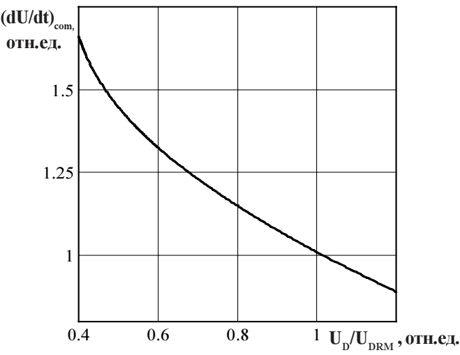
Рисунок 13 - Зависимость критической скорости нарастания коммутационного напряжения (dU Д /dt) com (отн.ед.) от величины приложенного напряжения U Д /U ДRМ (отн.ед.) при I Т = I ТRMS , T Г = 125 °С, t Г = 10 мс.
