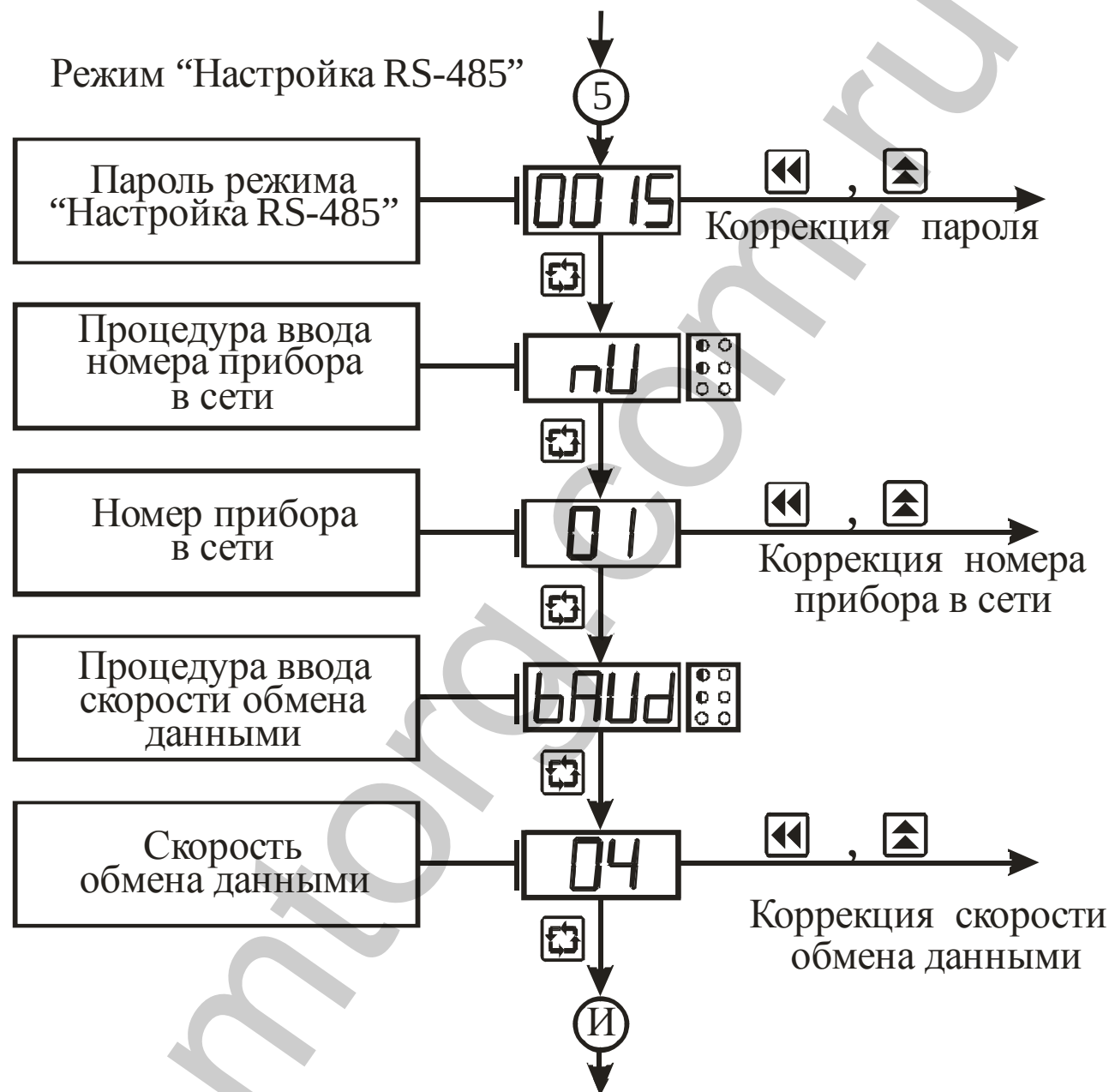
Рисунок 3.10 – Схема алгоритма работы в режиме "Настройка RS-485"
