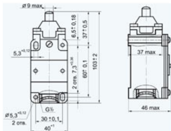
Рисунок А1 Выключатель ВП15К21А211
