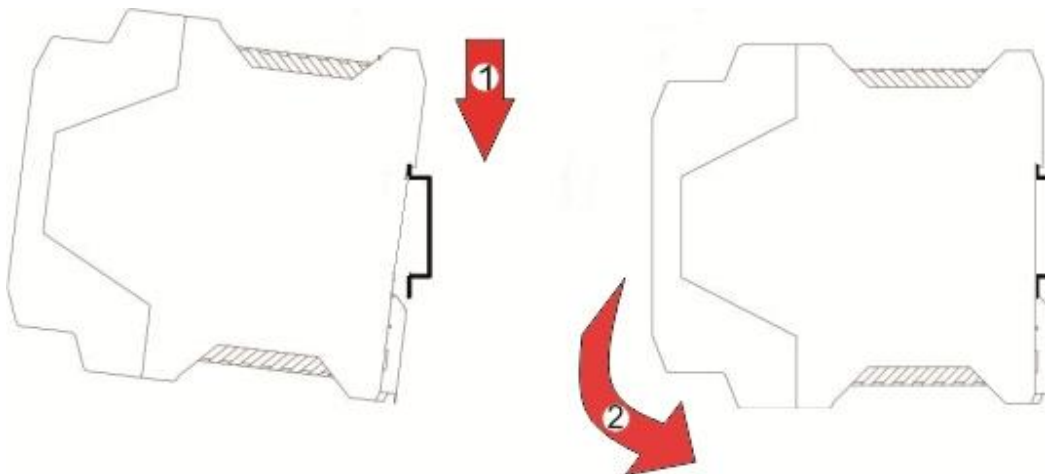
Рисунок 3.2 – Схема крепления преобразователя ПНС-101 на DIN-рельсе
