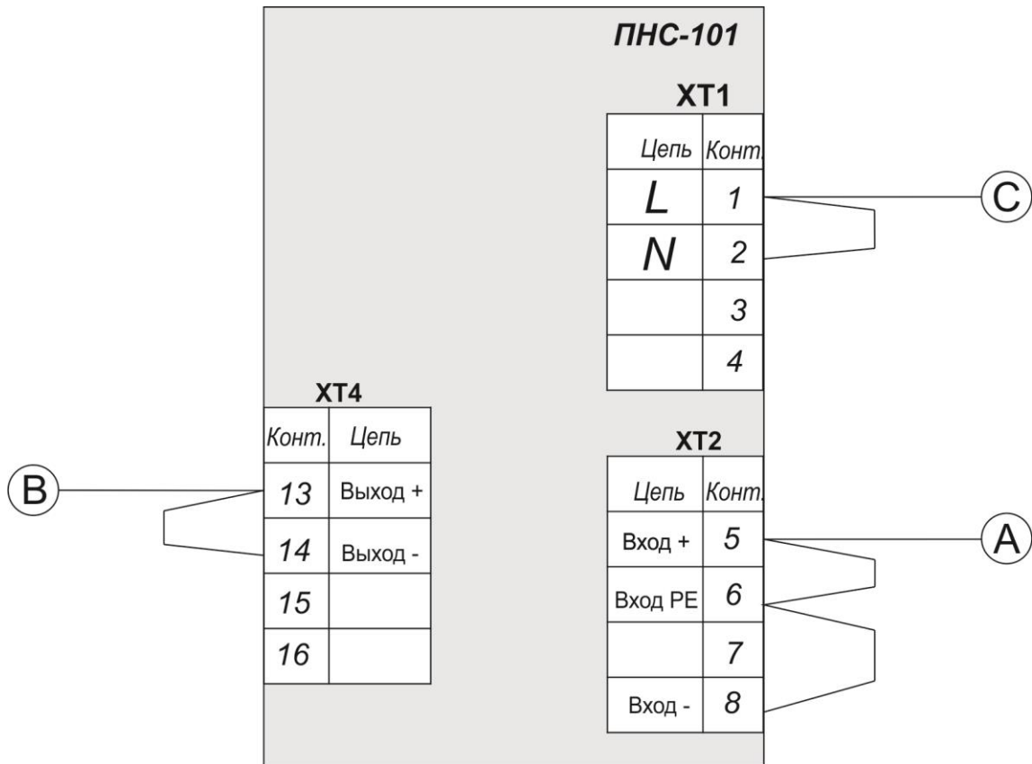
Рисунок Б.1 – Схема проверки сопротивления изоляции
