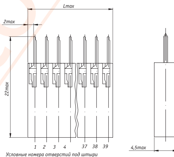
Рисунок 4 - Вилка ОНп-КГ-29
