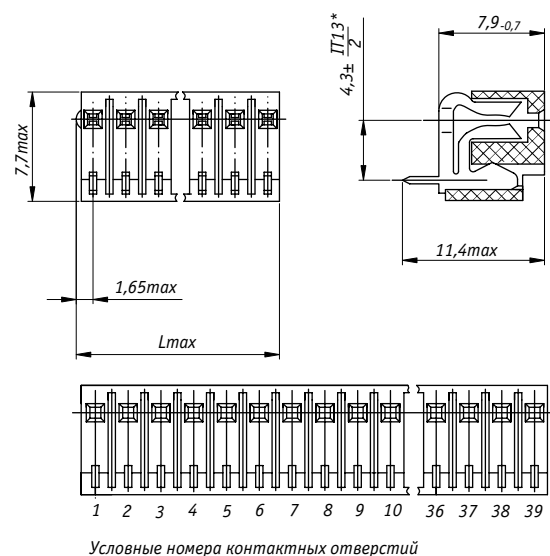
*Размеры для справок Рисунок 2 - Розетка ОНп-КГ-26 прямая
