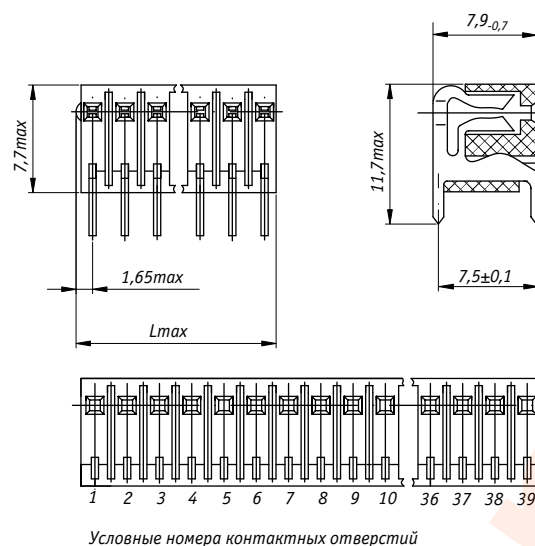
Рисунок 3 - Розетка ОНп-КГ-26 угловая
